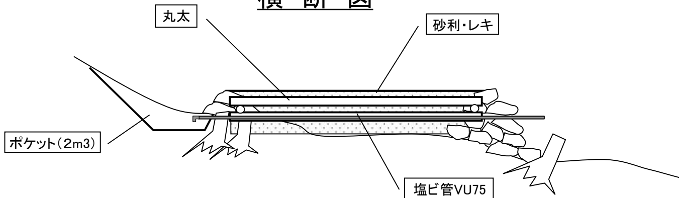
横断図
