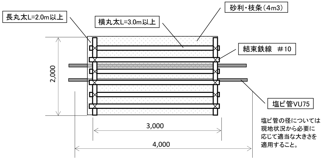
平面图
