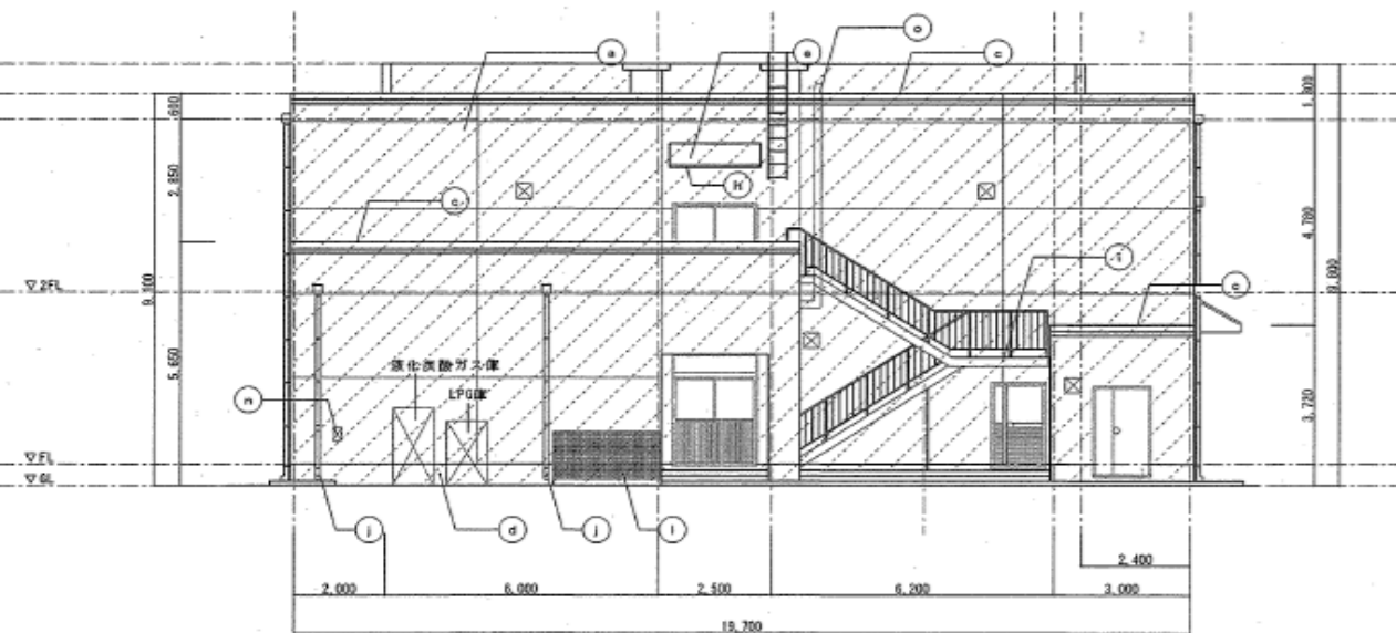
東立図 1/100
