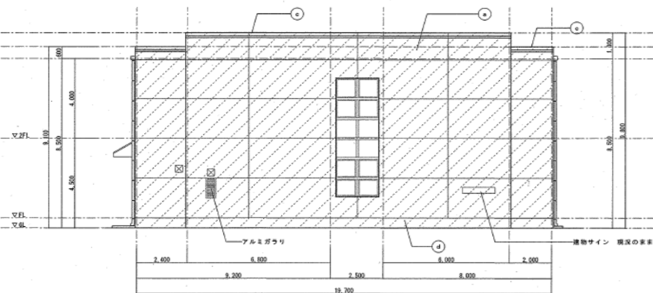
西立図 1/100
