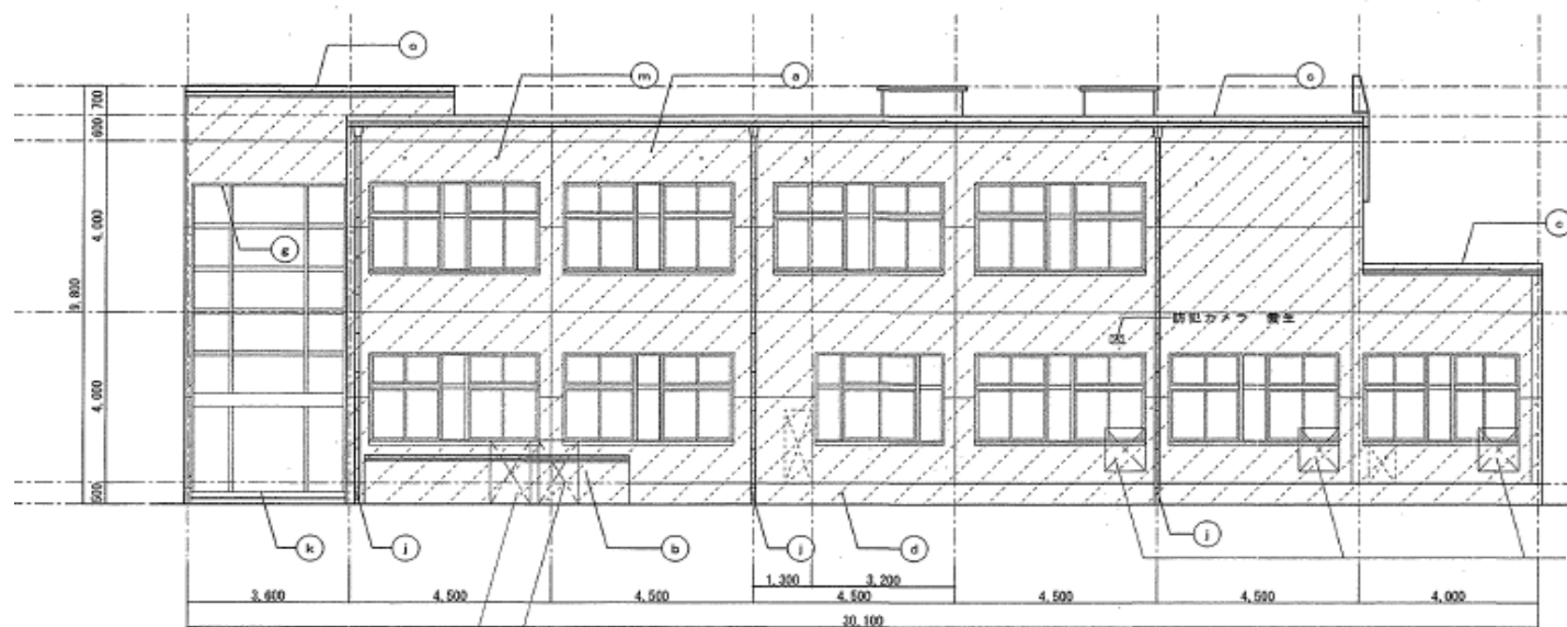
南立図 1/100
