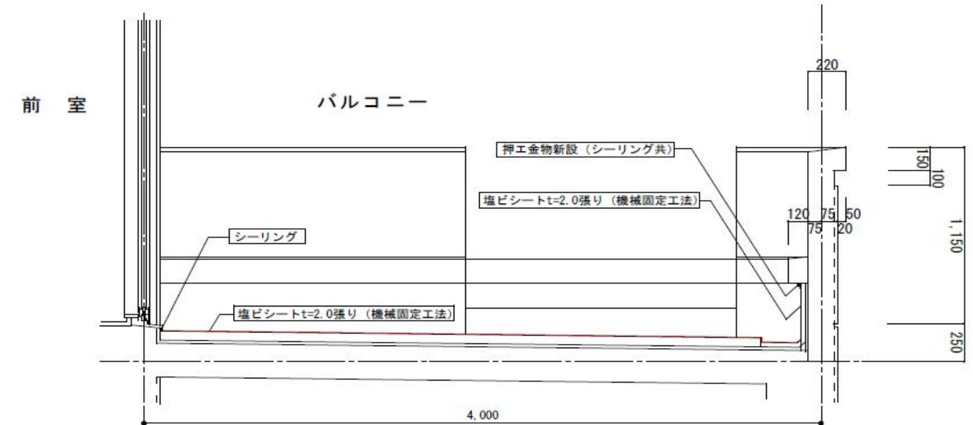
E-E' 断面図 (改修)
