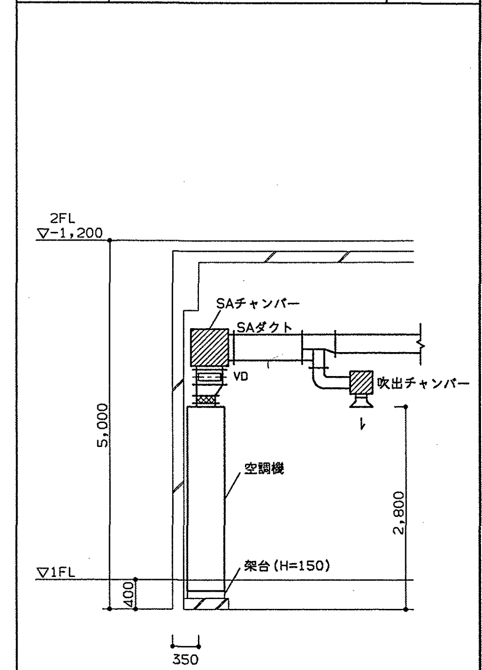
2 空調機まわり断面詳細図 1/50
