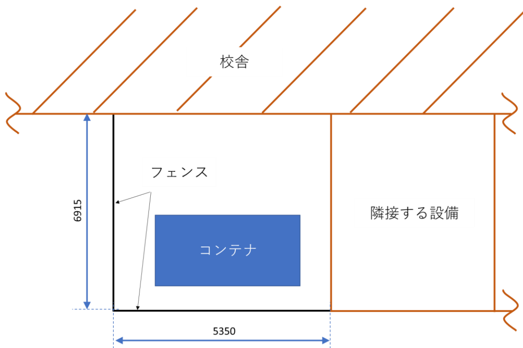
図1. フェンスの設置について
