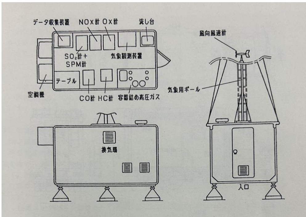
図4. 局舎の構造の例
