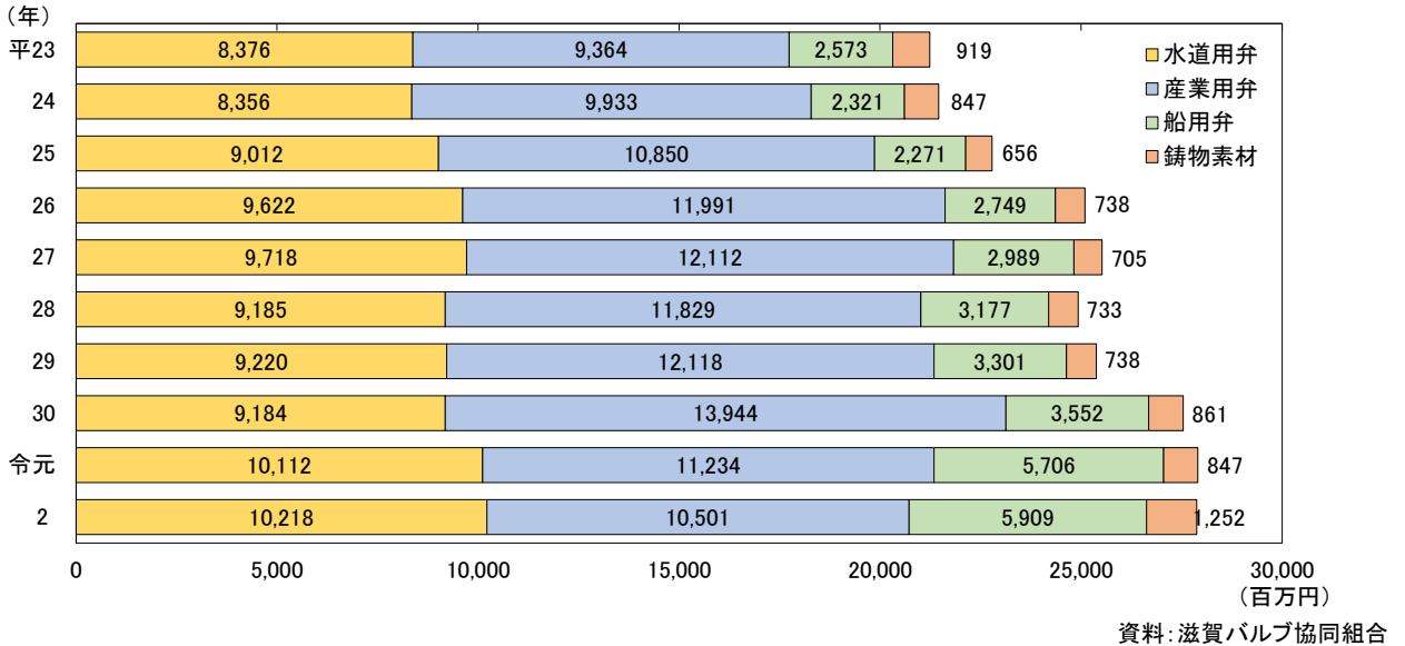
◆彦根バルブ産地 品種別生産額の推移(図3-7-3)
