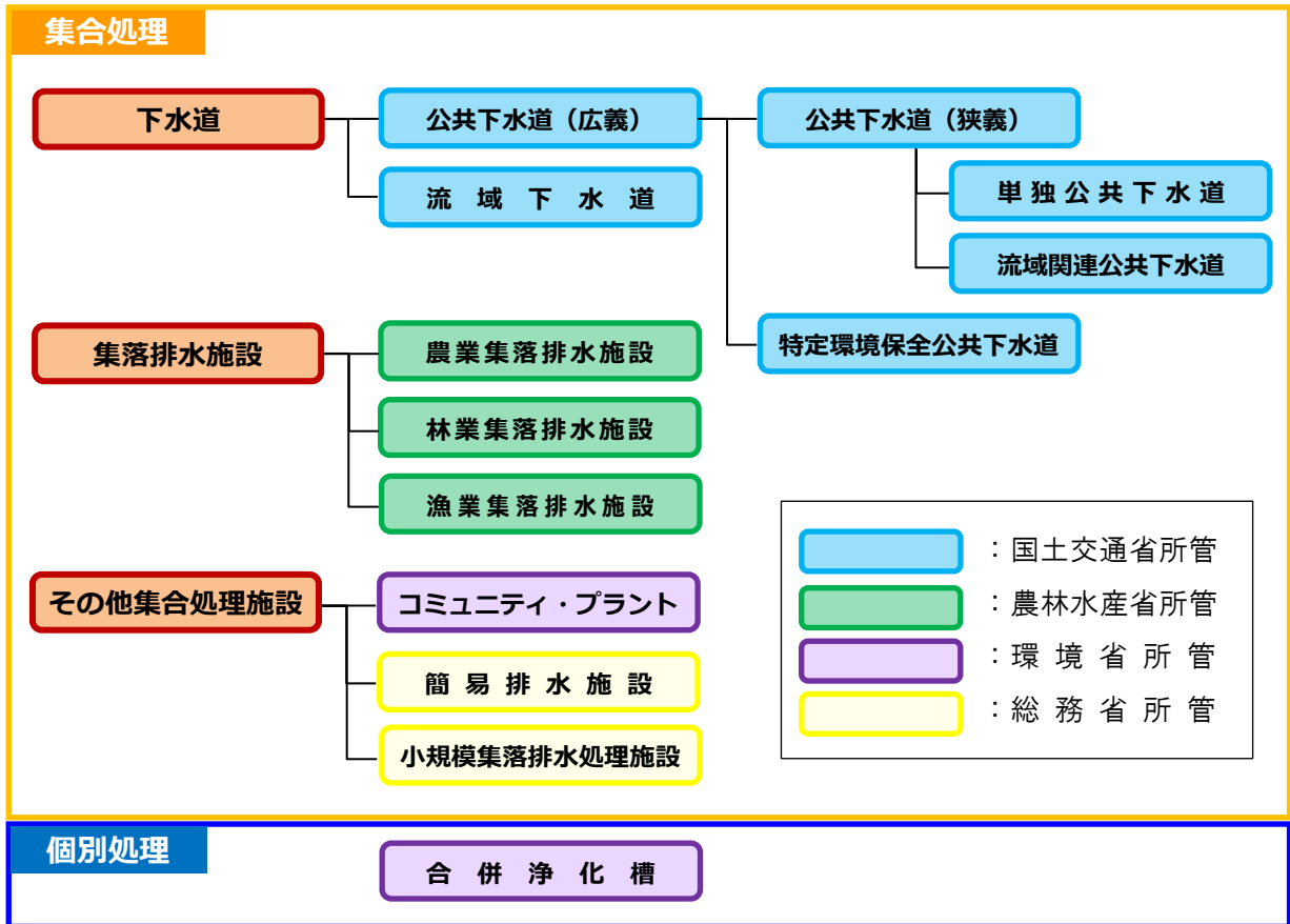
図 1 汚水処理施設の種類
