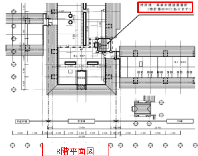
付近見取り図・配置図・R階平面図
