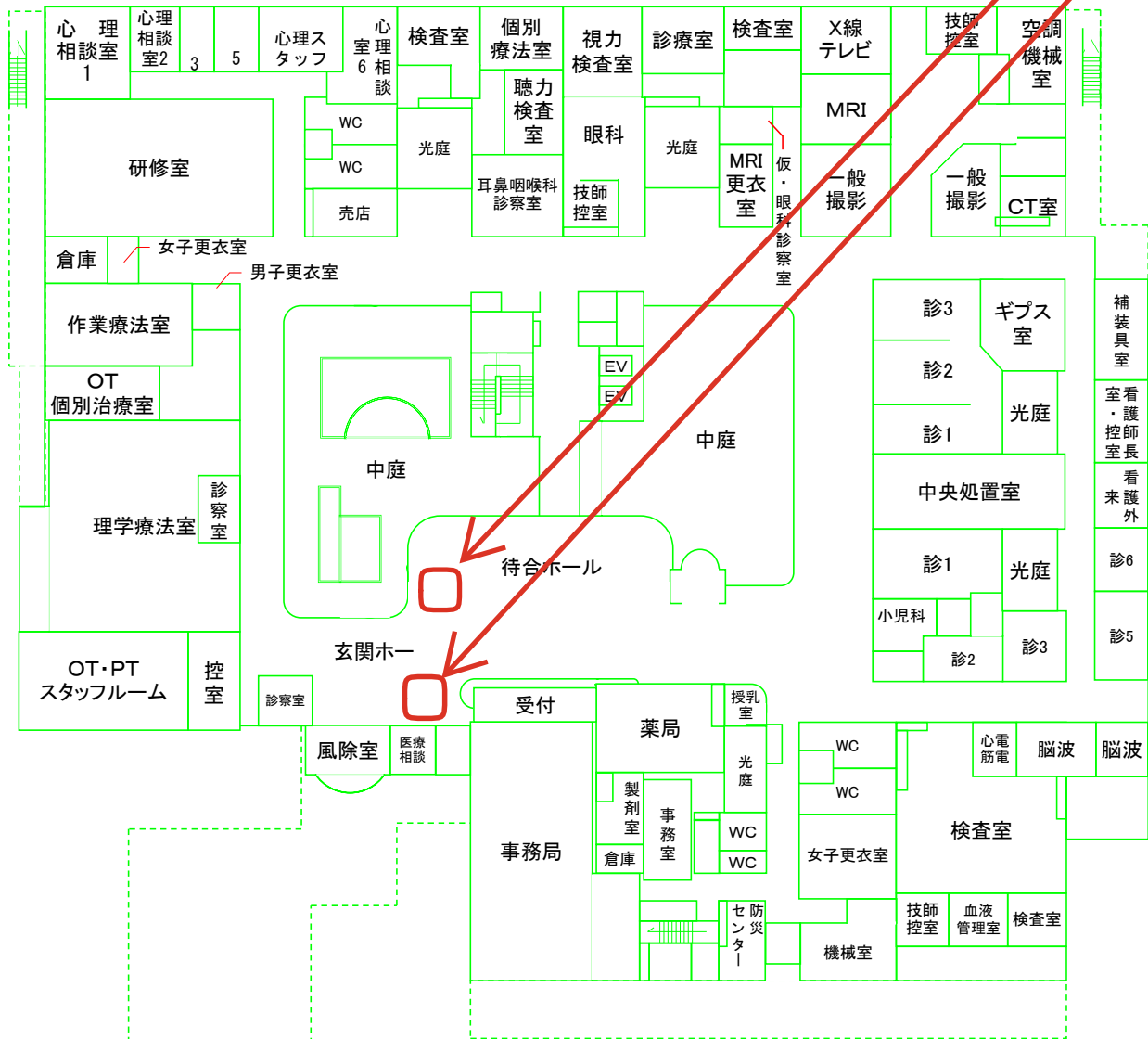
【地階平面図】
