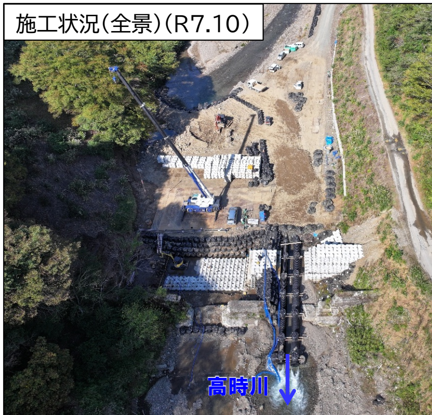
施工状況(R7.10)
