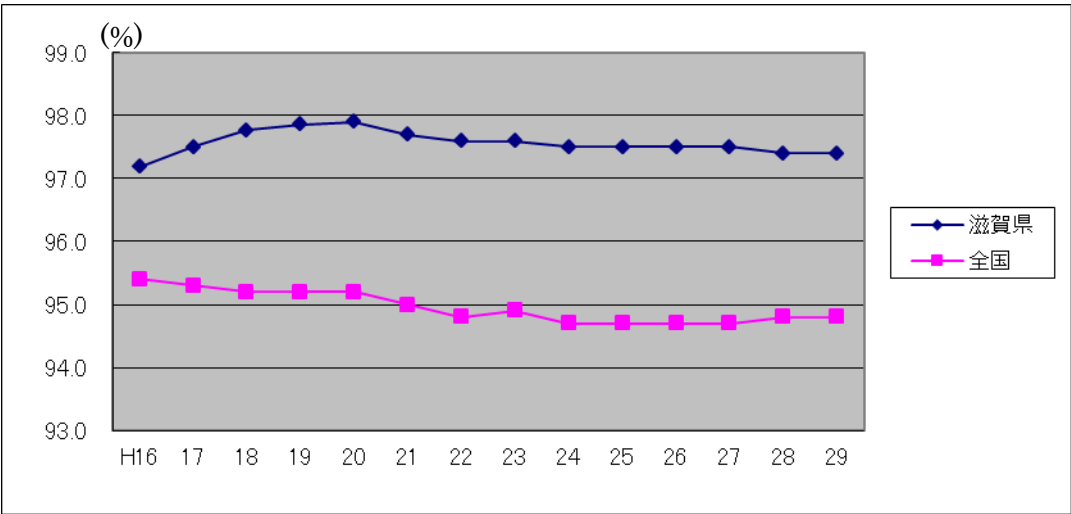
図 3 性比の推移
