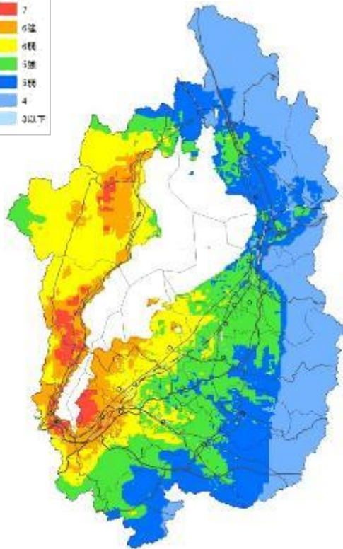
18 震度分布図
