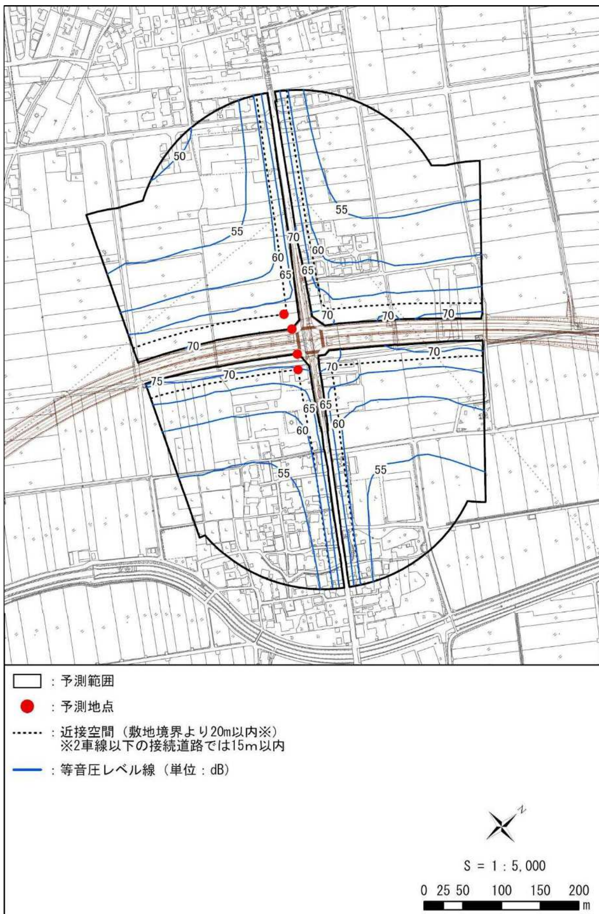
図 11-2-17(21) 自動車の走行に係る騒音分布図 (D①：愛荘町市（昼間/地上 1.2m）)
