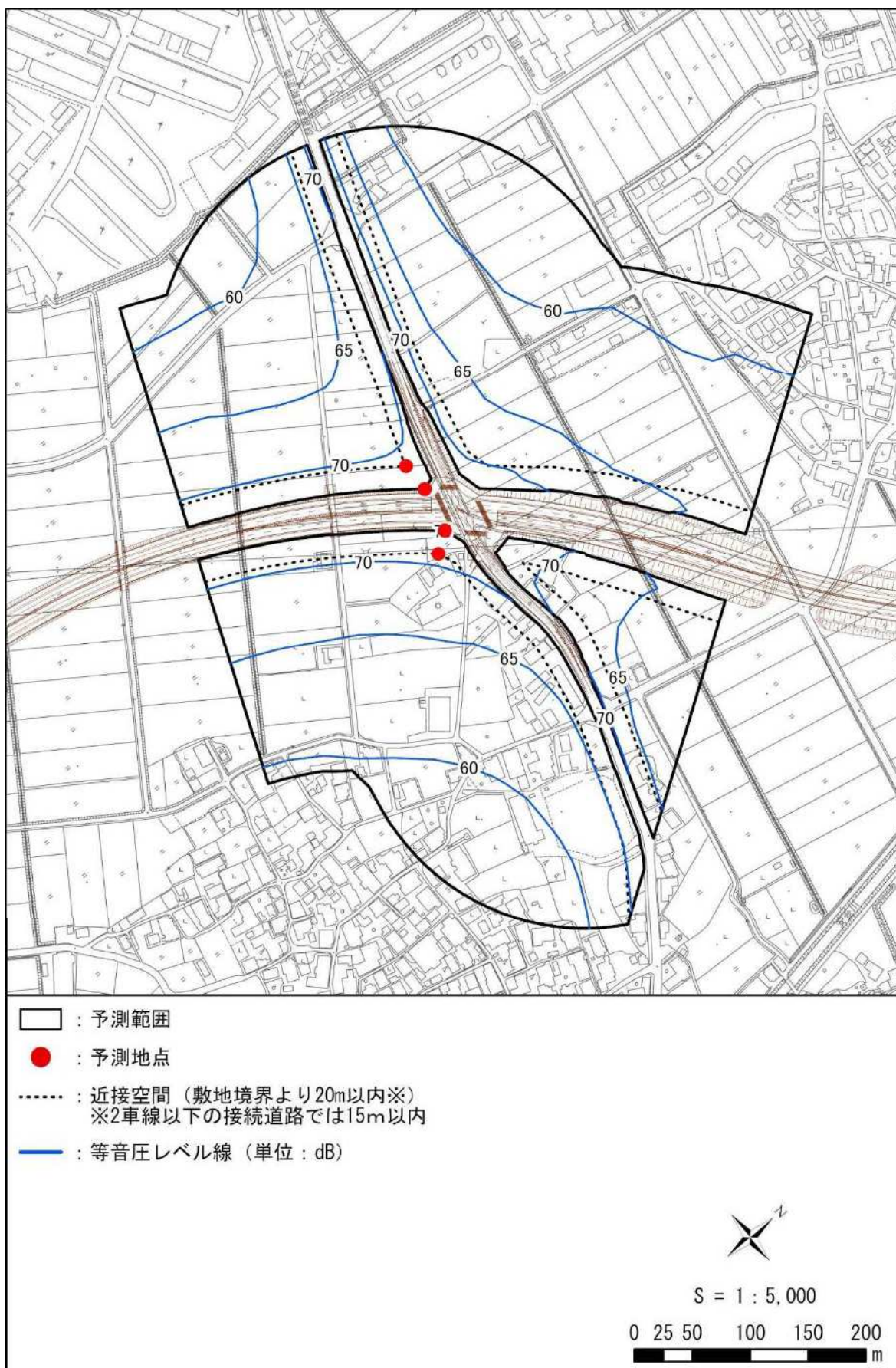
図 11-2-17(26) 自動車の走行に係る騒音分布図 (D③：愛荘町東円堂(2)（昼間/地上 4.2m）)
