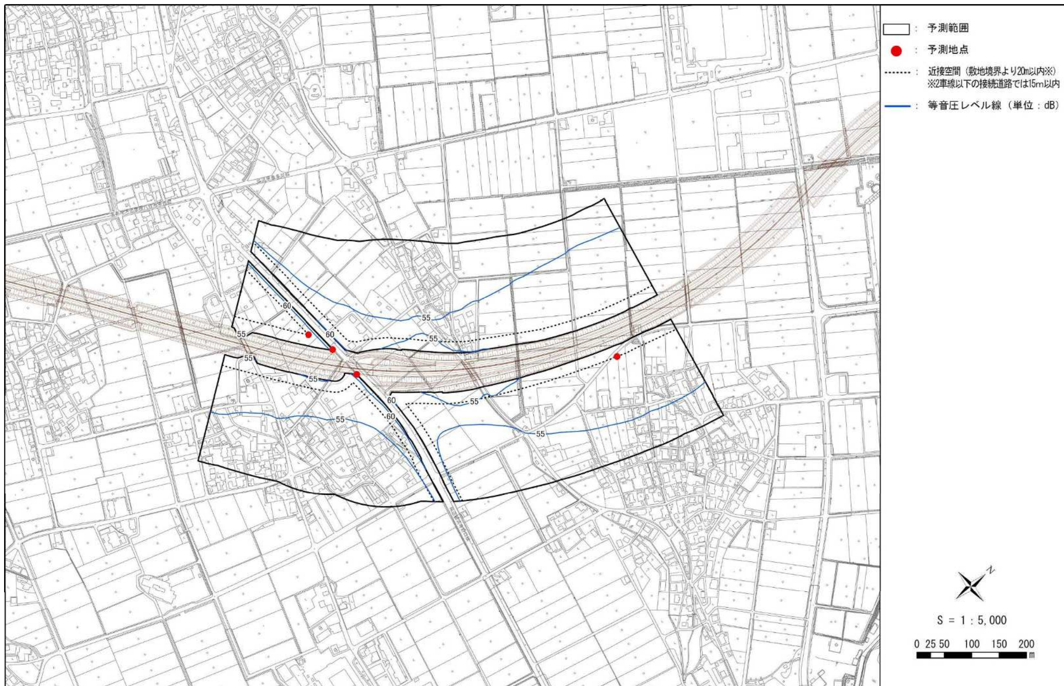
図 11-2-17(11) 自動車の走行に係る騒音分布図（C①：甲良町横関（夜間/地上1.2m））
