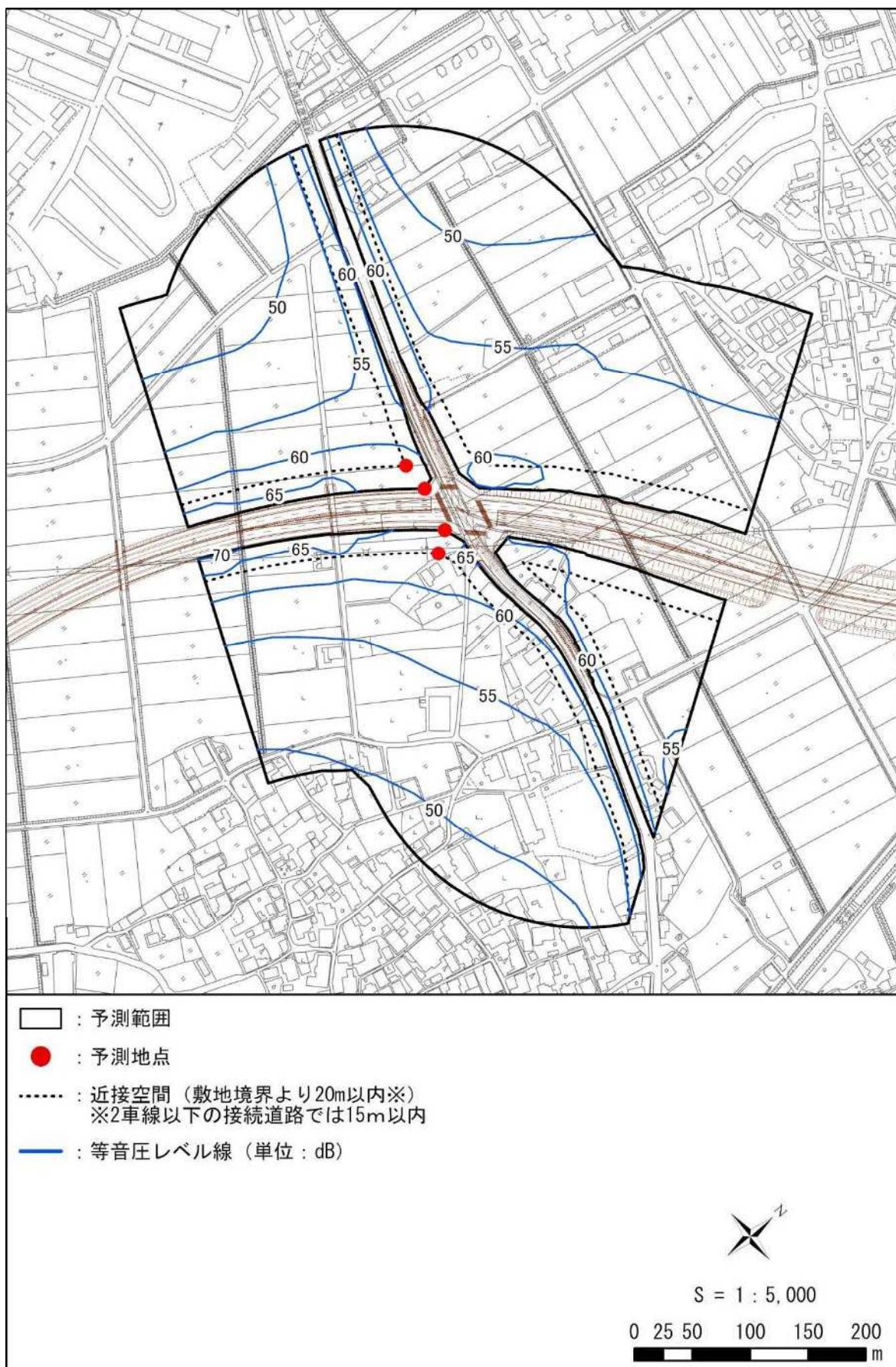
図 11-2-17(27) 自動車の走行に係る騒音分布図 (D③：愛荘町東円堂(2)（夜間/地上1.2m）)
