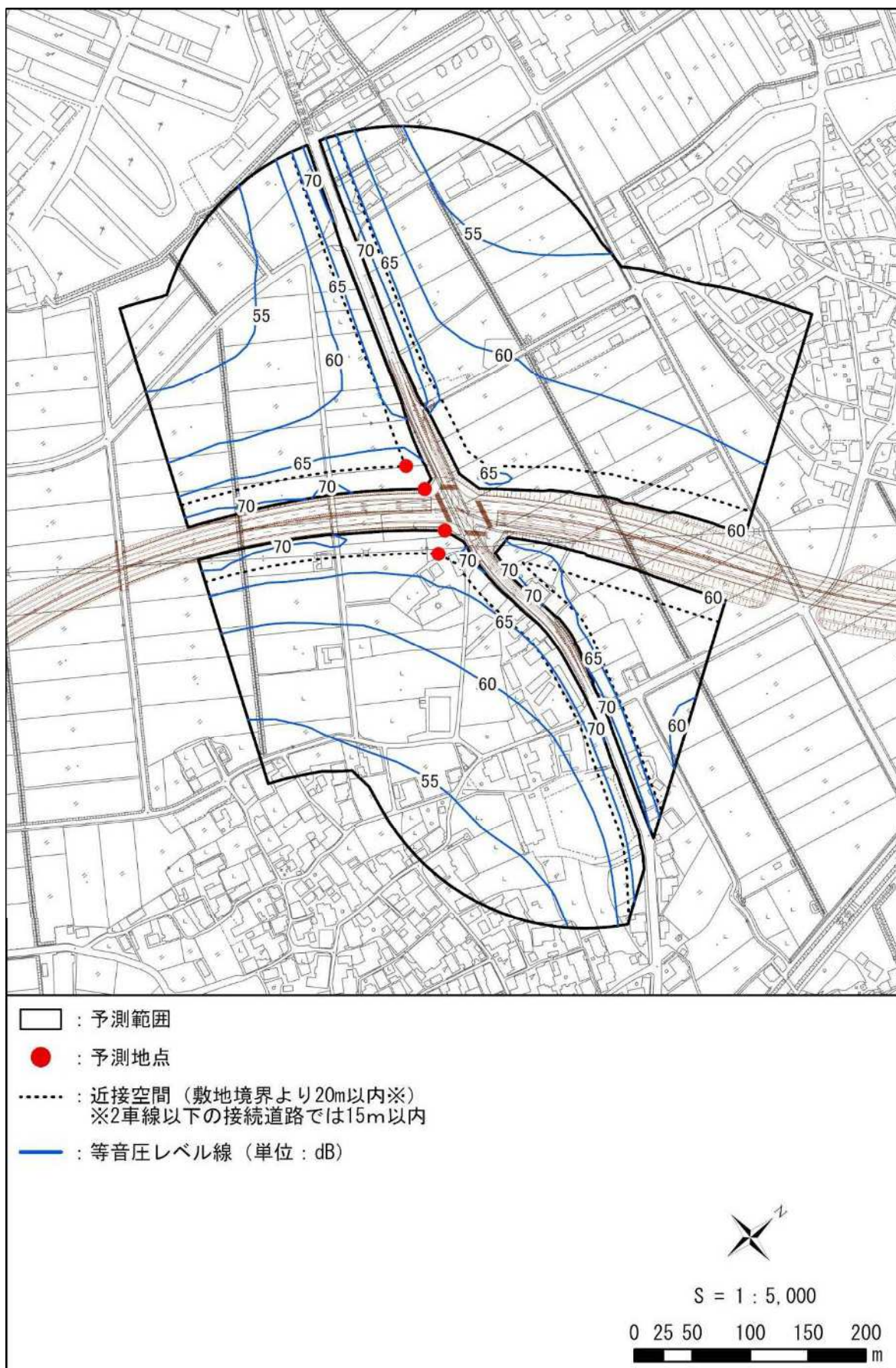
図 11-2-17(25) 自動車の走行に係る騒音分布図 (D③：愛荘町東円堂(2)（昼間/地上 1.2m）)
