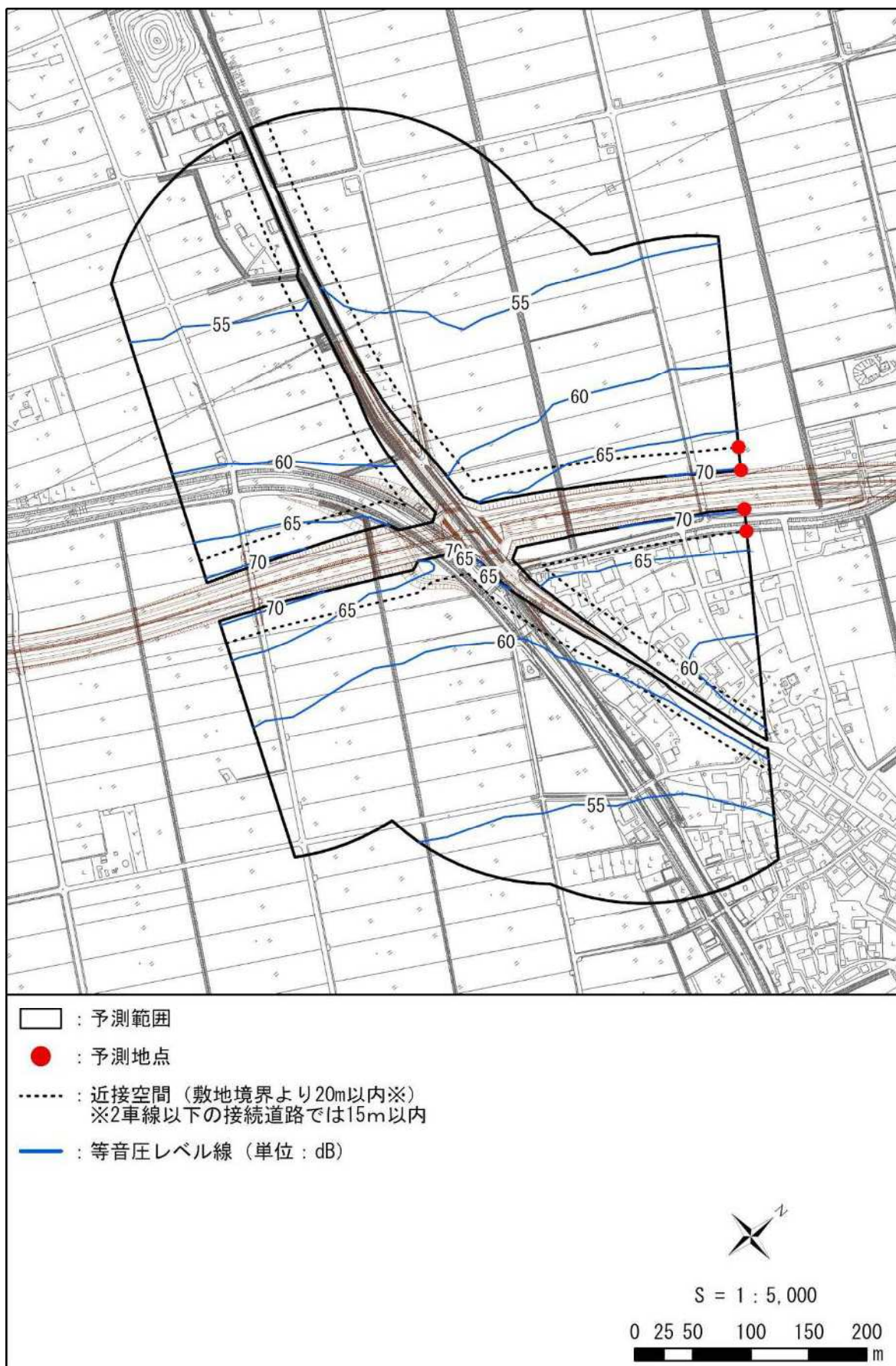
図 11-2-17(20) 自動車の走行に係る騒音分布図（C③：豊郷町雨降野（夜間/地上 4.2m））
