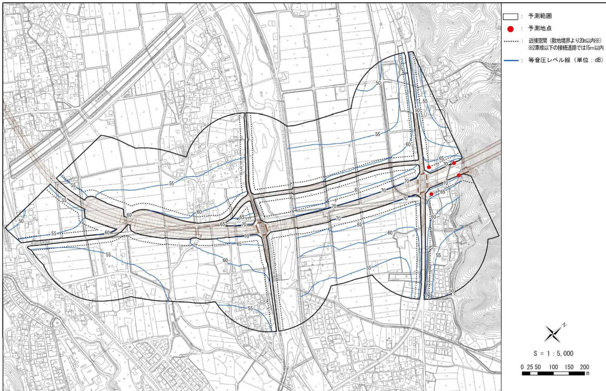
図 11-2-17(8) 自動車の走行に係る騒音分布図 (B①: 多賀町木曾 (夜間/地上 4.2m))
