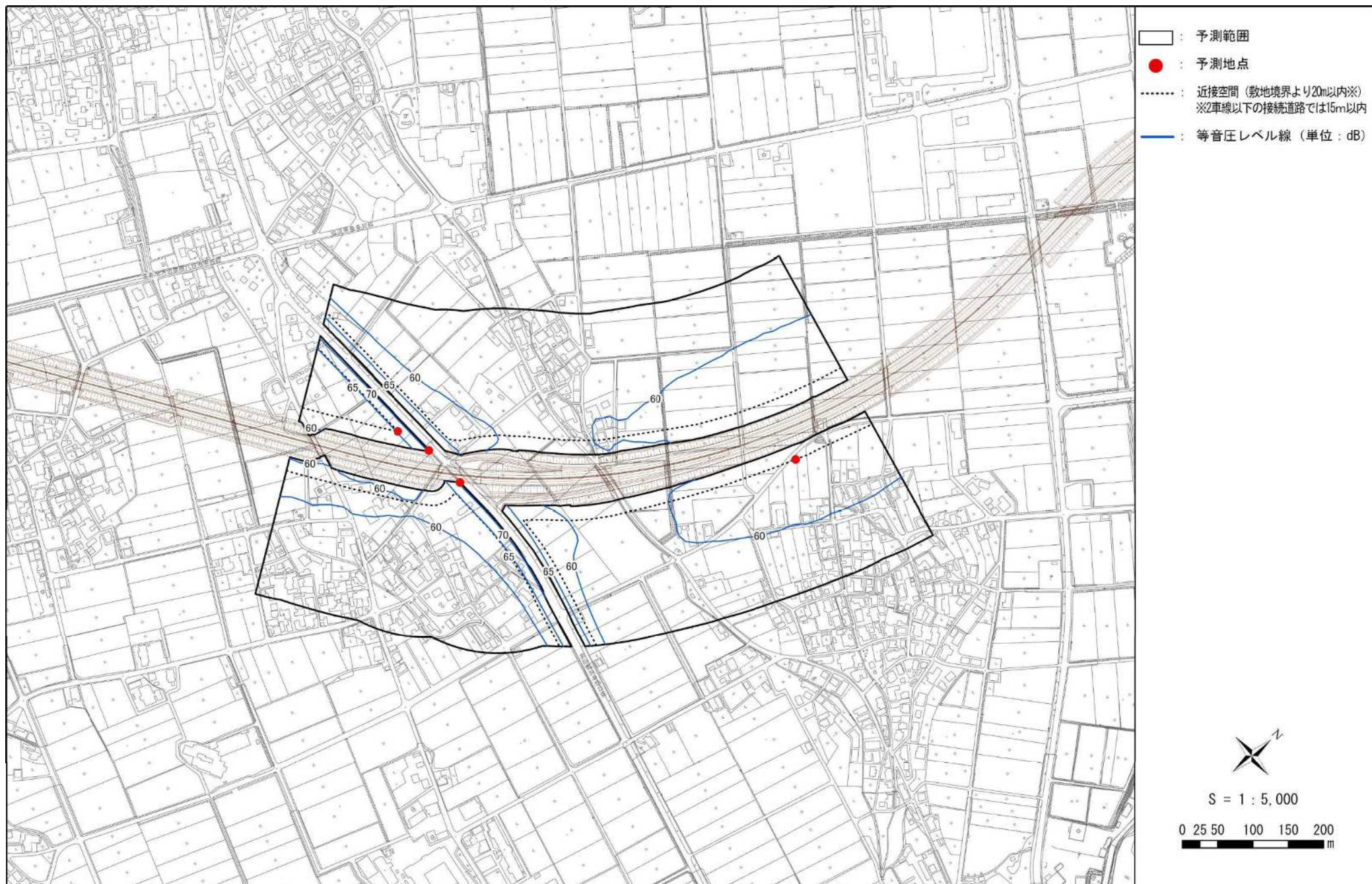
図 11-2-17(9) 自動車の走行に係る騒音分布図（C①：甲良町横関（昼間/地上1.2m））
