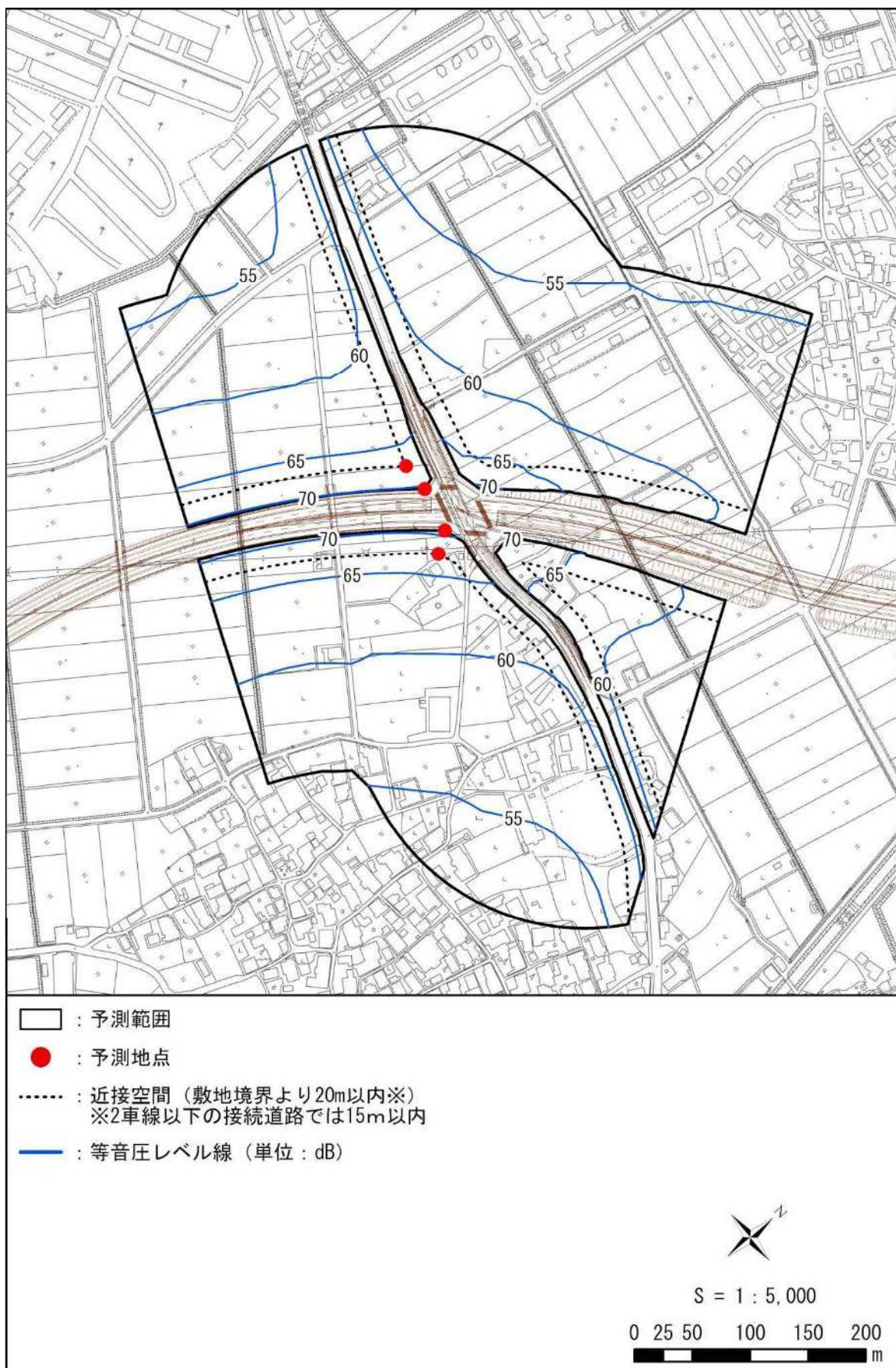
図 11-2-17(28) 自動車の走行に係る騒音分布図 (D③：愛荘町東円堂(2)（夜間/地上 4.2m）)
