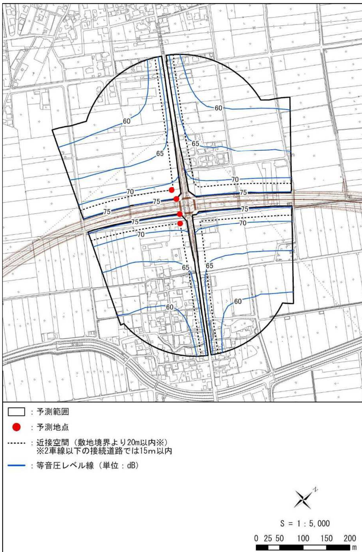
図 11-2-17(22) 自動車の走行に係る騒音分布図 (D①：愛荘町市（昼間/地上 4.2m）)
