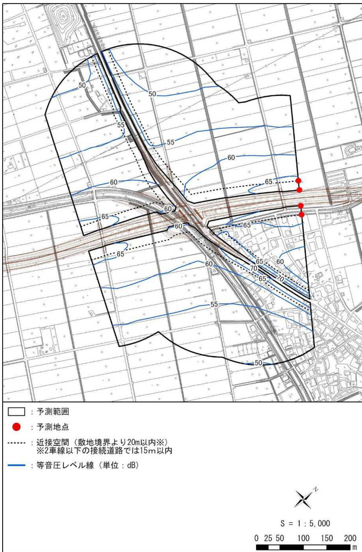
図 11-2-17(17) 自動車の走行に係る騒音分布図（C③：豊郷町雨降野（昼間/地上1.2m））
