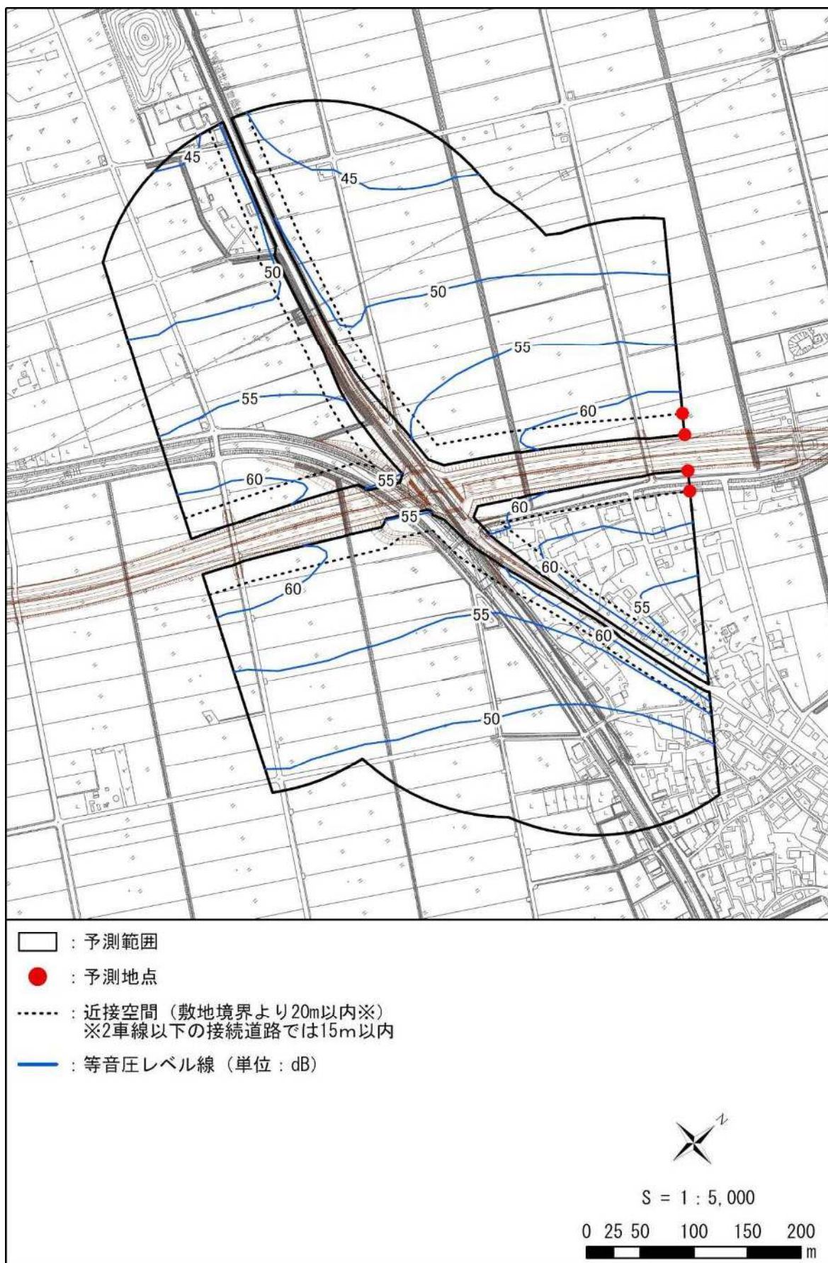
図 11-2-17(19) 自動車の走行に係る騒音分布図（C③：豊郷町雨降野（夜間/地上1.2m））
