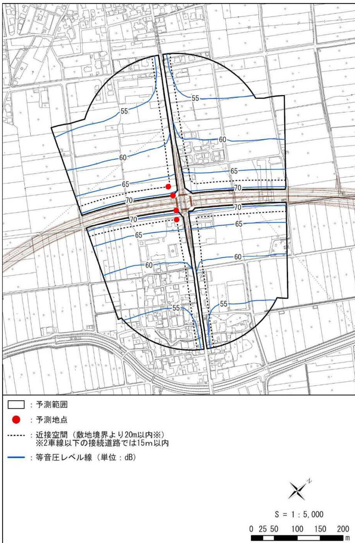
図 11-2-17(24) 自動車の走行に係る騒音分布図 (D① : 愛荘町市 (夜間/地上 4.2m))
