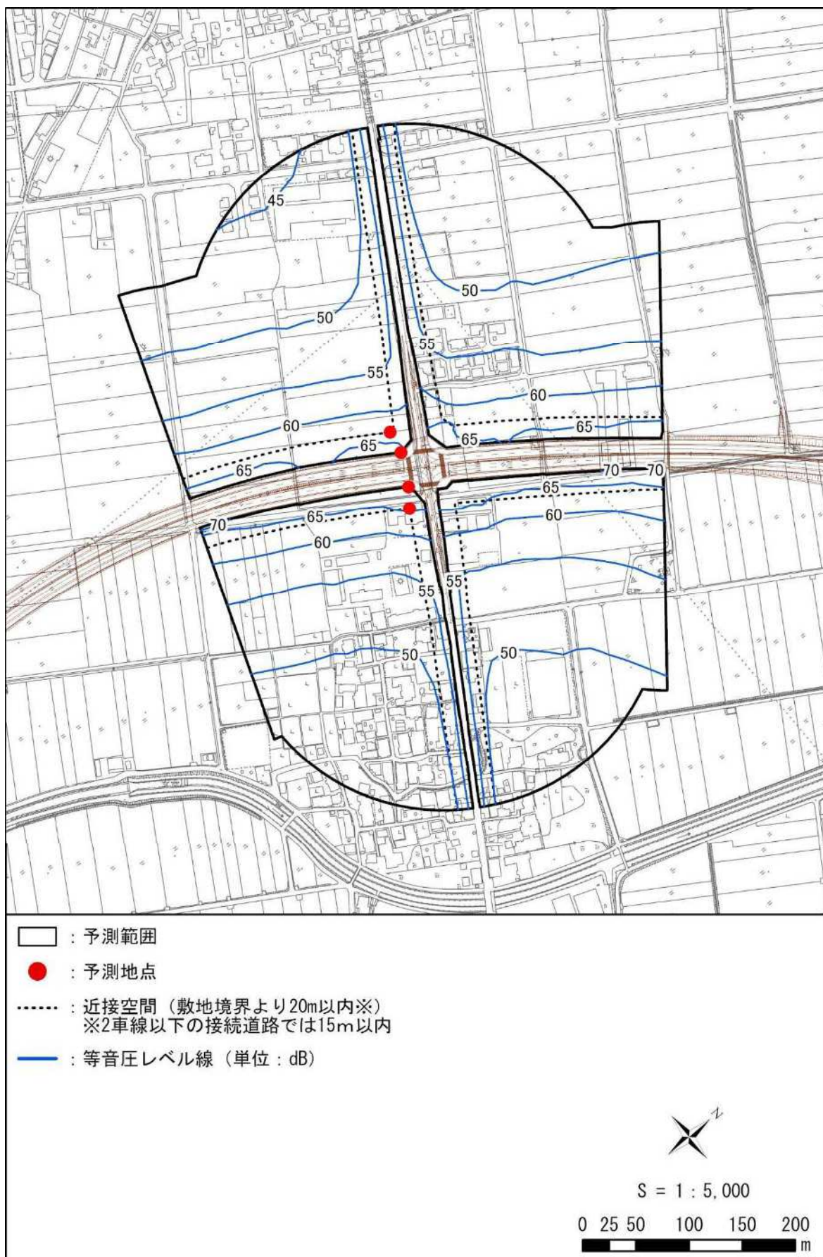
図 11-2-17(23) 自動車の走行に係る騒音分布図 (D①：愛荘町市（夜間/地上 1.2m）)
