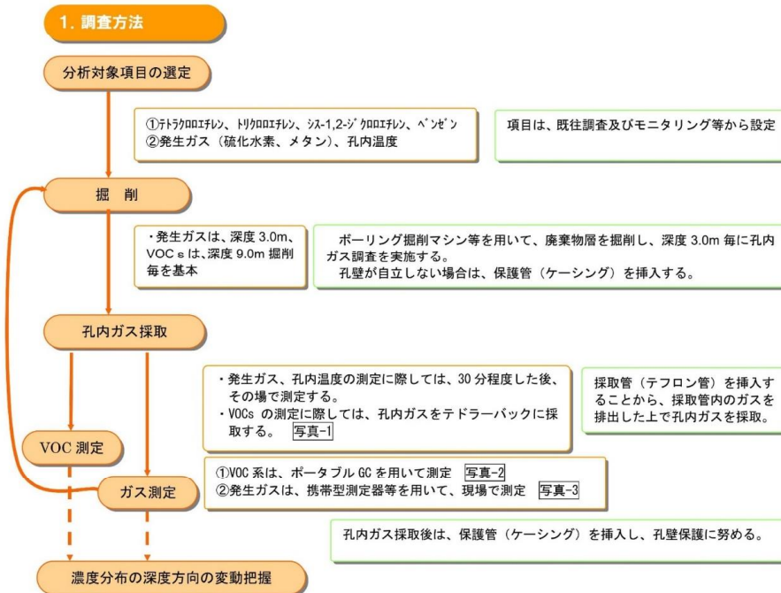
図-2.2.1 孔内ガス調査フロー
