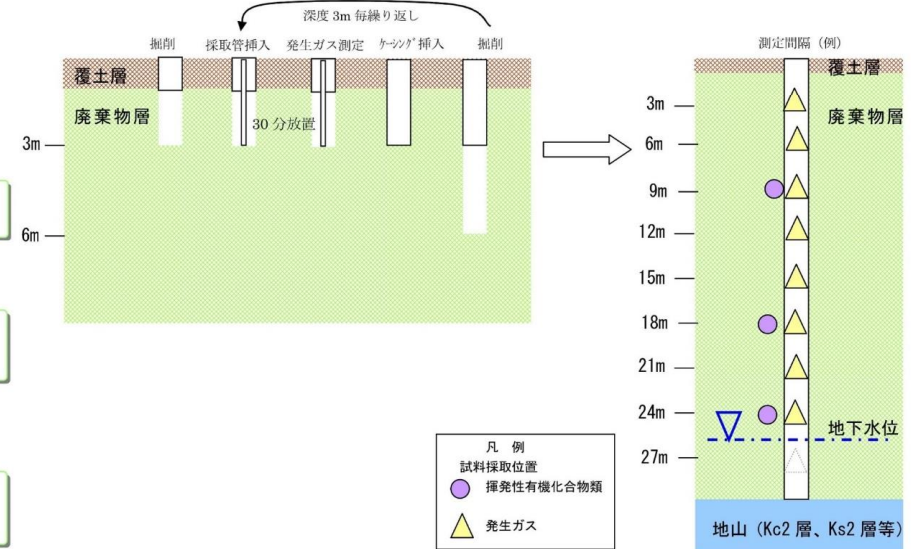
図-2.2.2 廃棄物分析試料採取の方法
