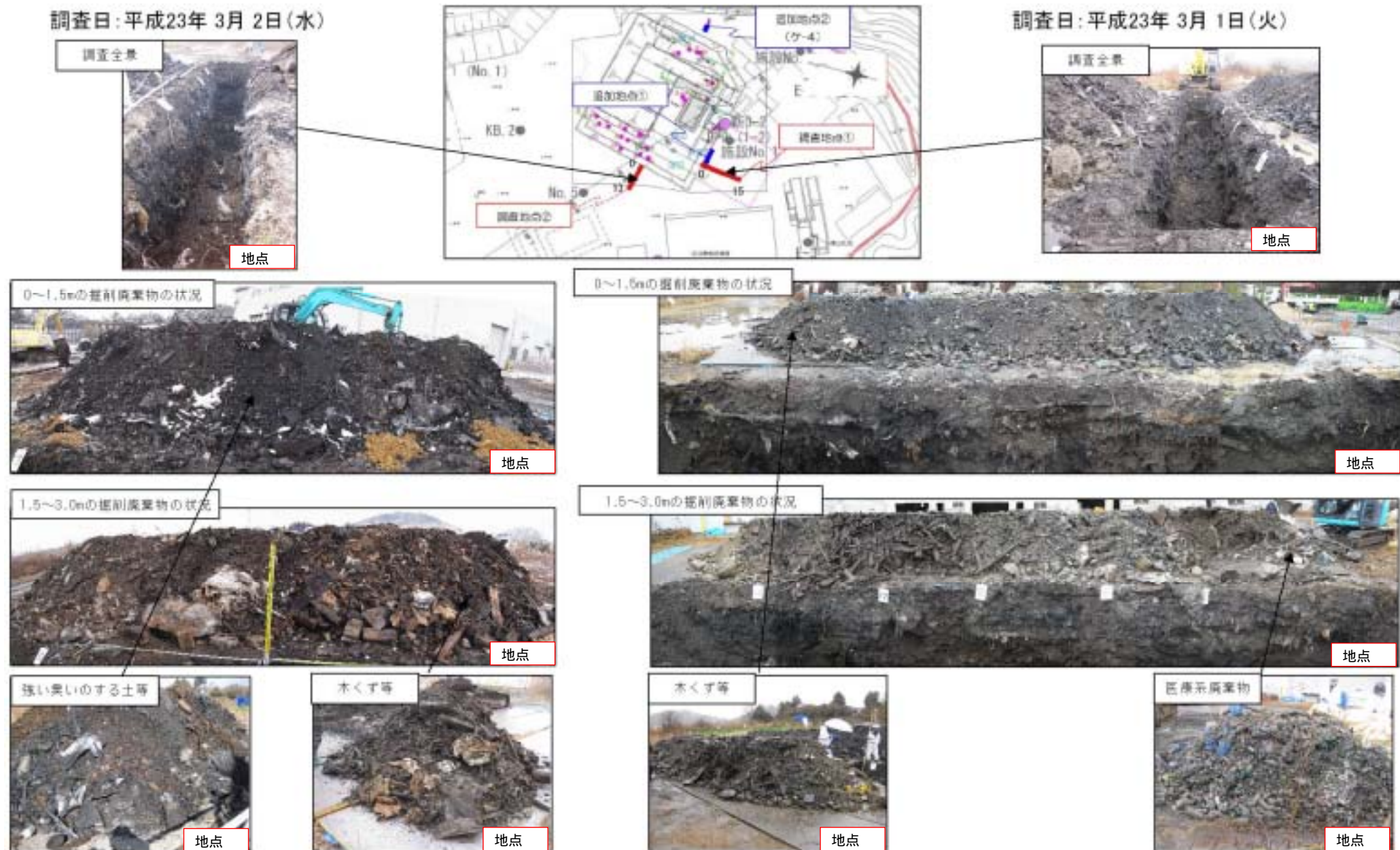
写真-3.2.2 各試掘箇所の掘削状況
