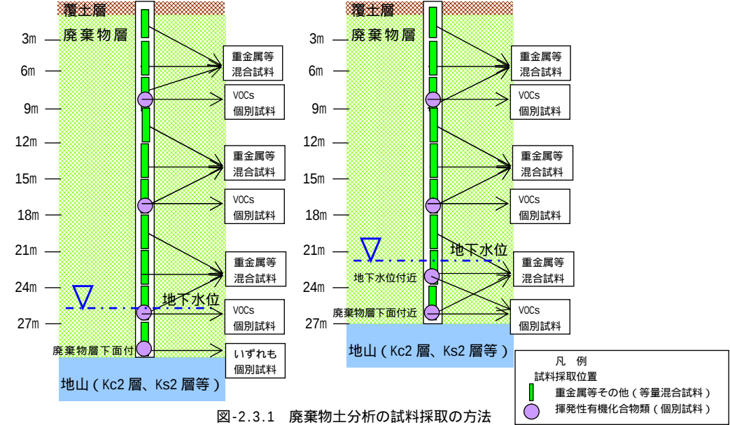
図-2.3.1 廃棄物土分析の試料採取の方法
