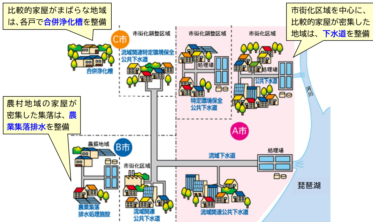
図 1 污水处理施設の種類
