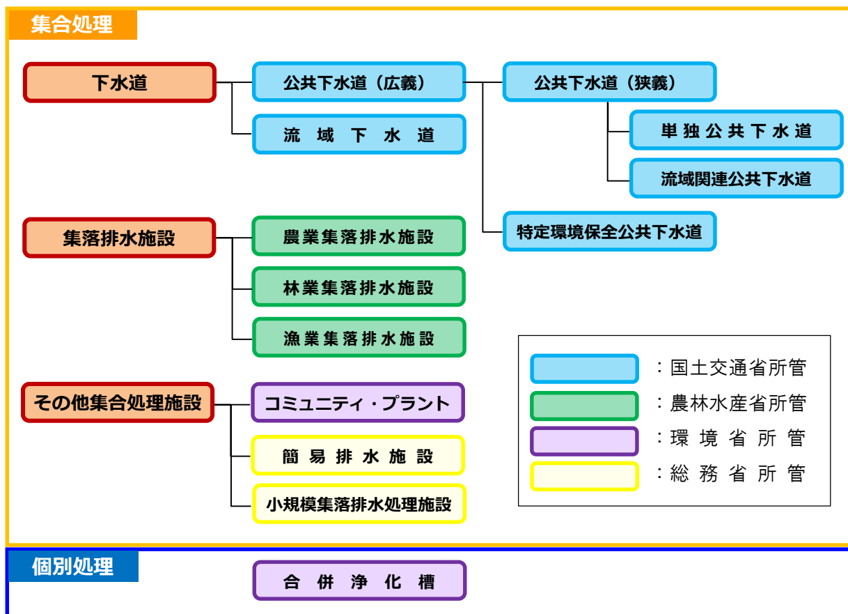
図 1 污水处理施設の種類
