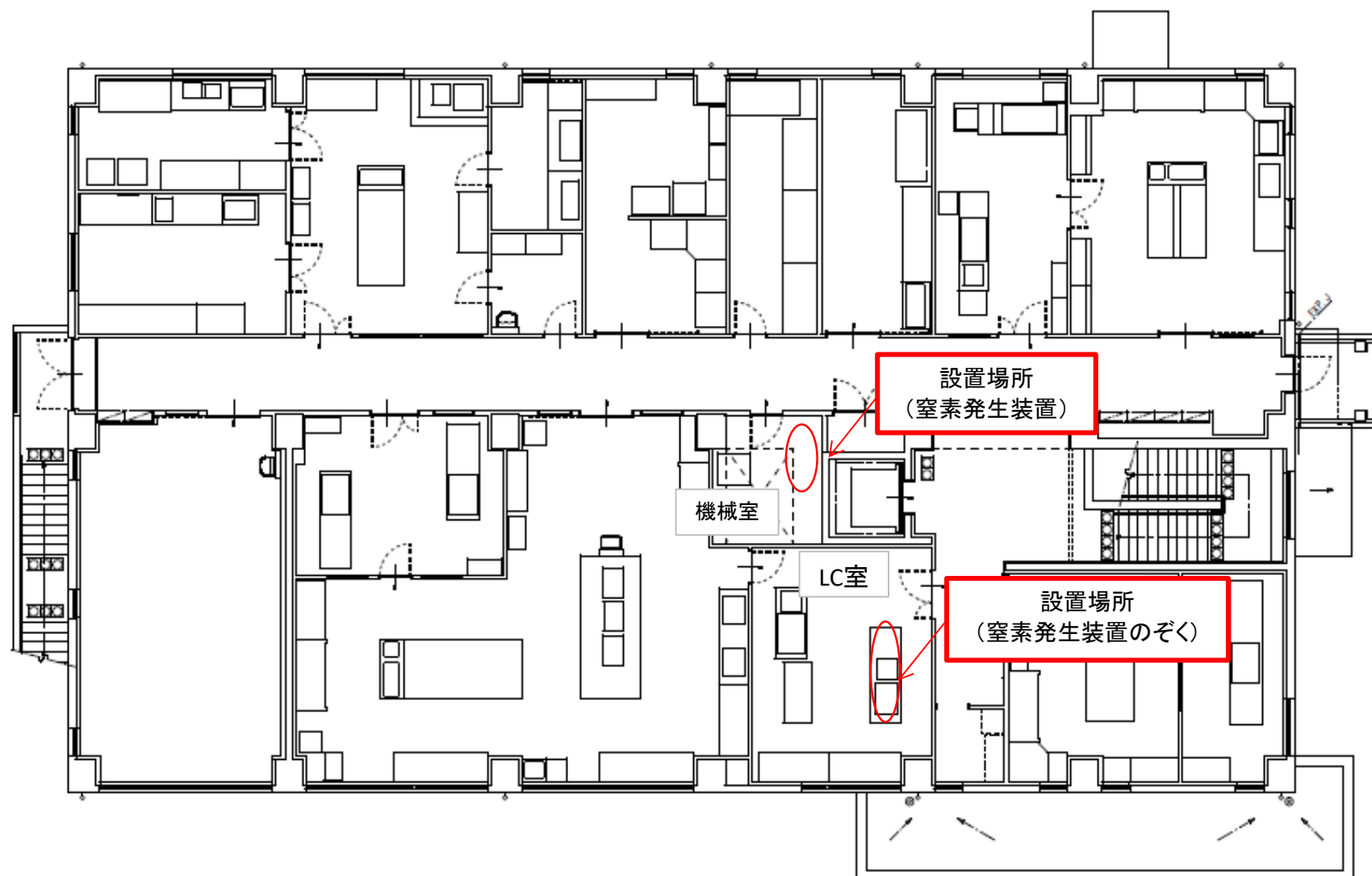
平面図 水質試験棟 2F
