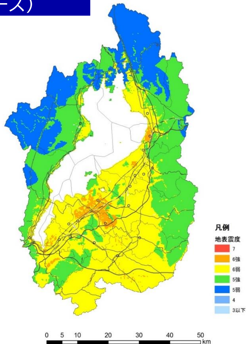
地表震度 南海トラフ陸側ケース-重ね合わせ最大値
