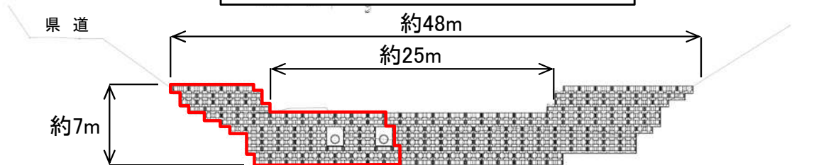
整備内容(横断図)＜上流面＞
