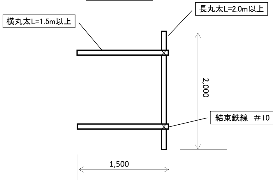
平 面 図
