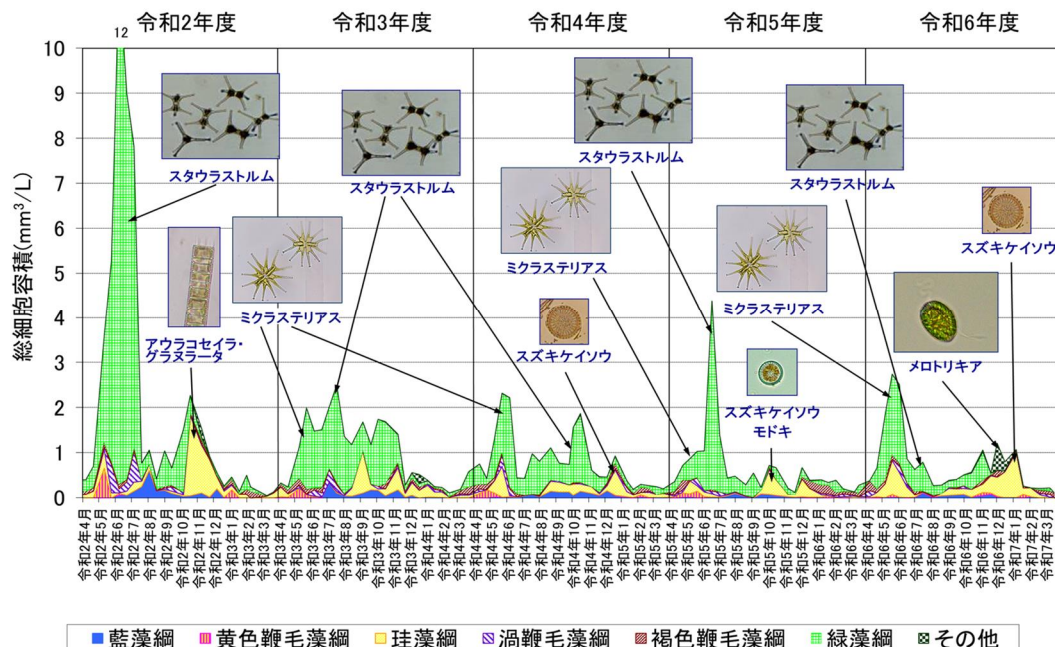
北湖における 植物プランクトン総細胞容積の変動(今津沖中央0.5m層,令和2年4月～令和7年3月)
