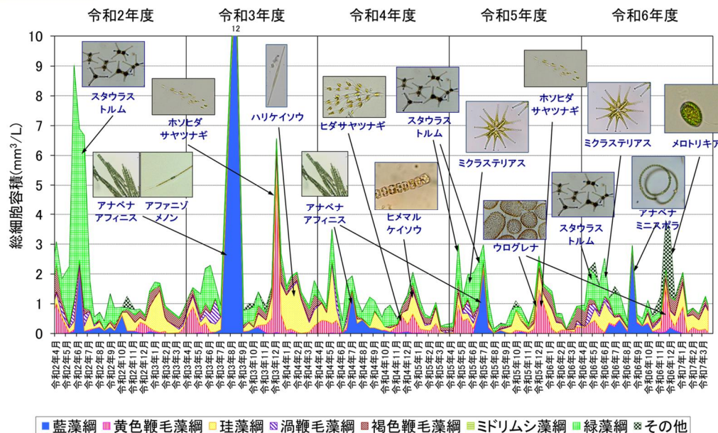
南湖における 植物プランクトン総細胞容積の変動(唐崎沖中央0.5m層,令和2年4月～令和7年3月)
