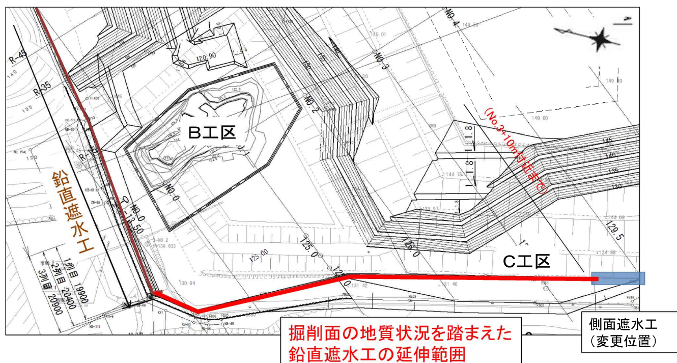
C工区付近概略平面図
