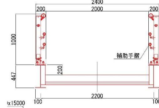
階段断面図
