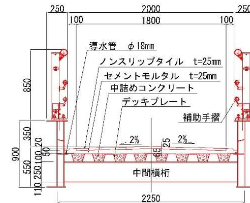
通路部標準断面図
