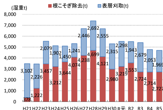
水草刈取除去量 推移 県全体
