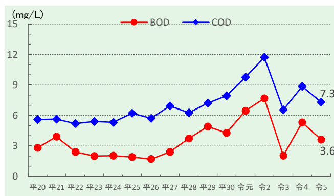
西の湖BOD・COD経年変化
