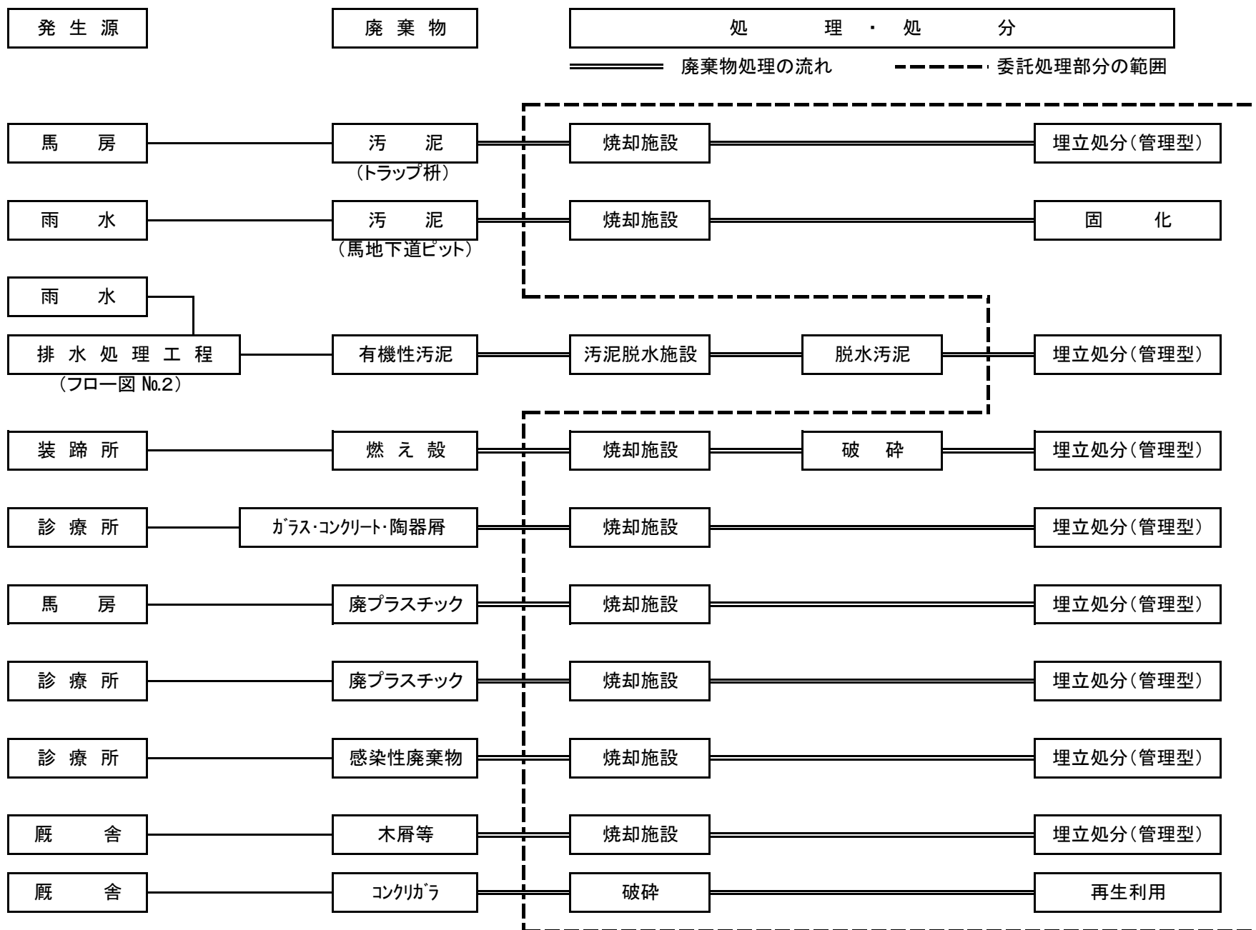
廃棄物処理フロー図(現状) No.1
