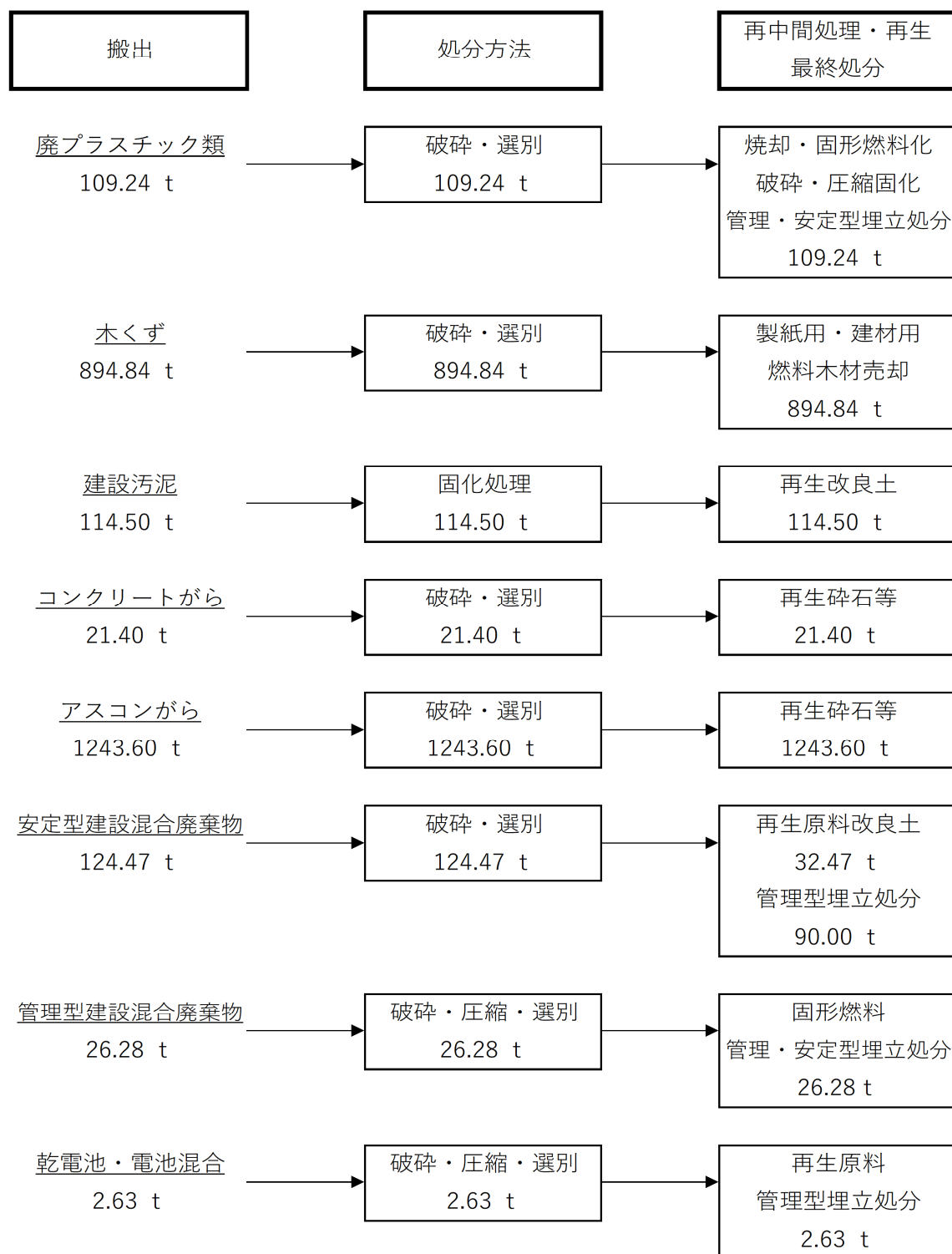
産業廃棄物処理工程表
