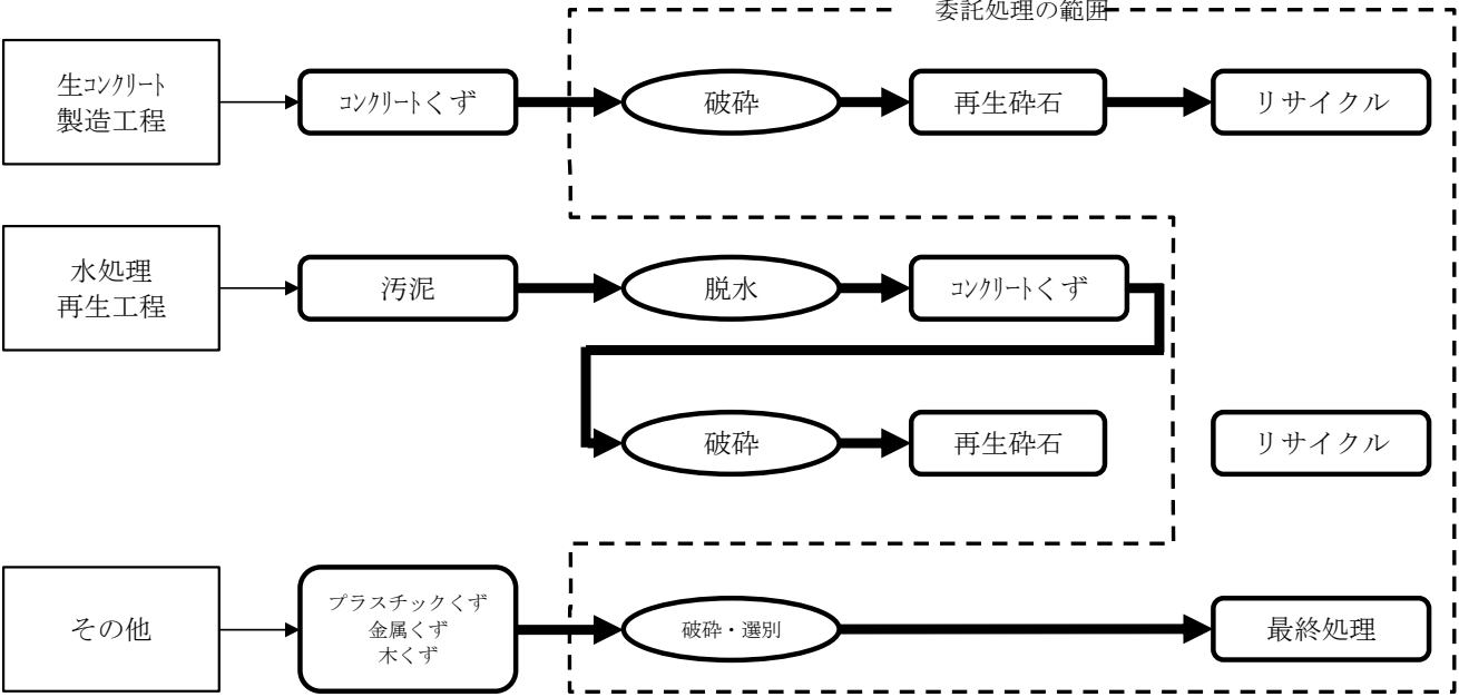
別紙 産業廃棄物の一連の処理の工程
