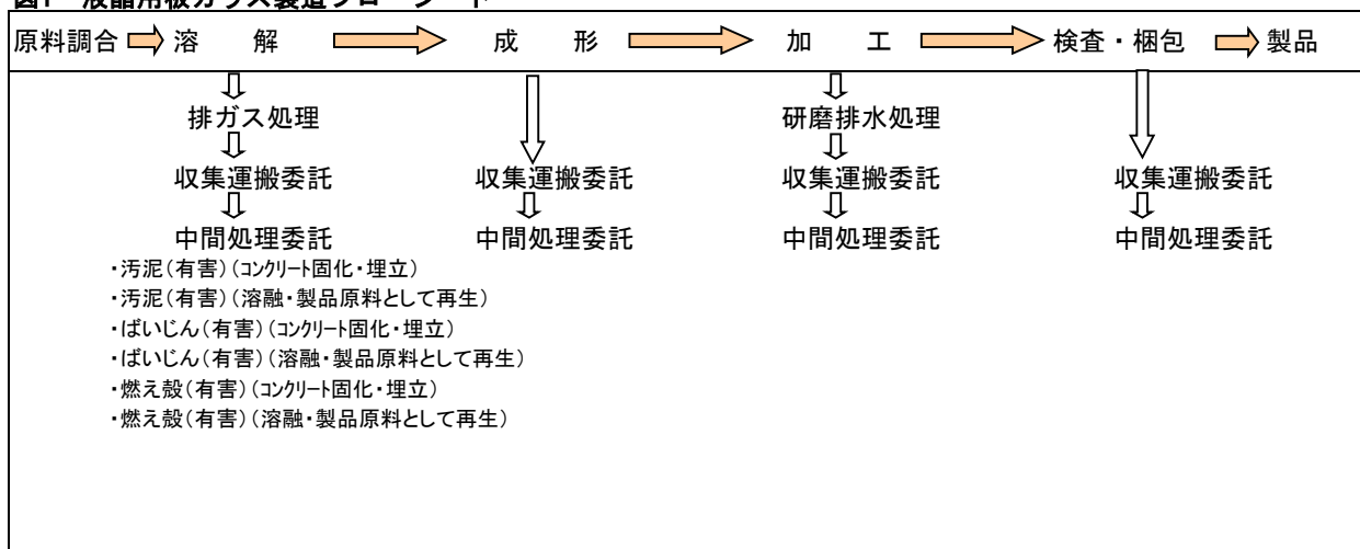
図1 液晶用板ガラス製造フローシート
