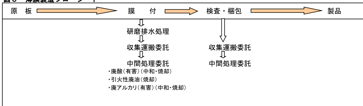
図3 薄膜製造フローシート
