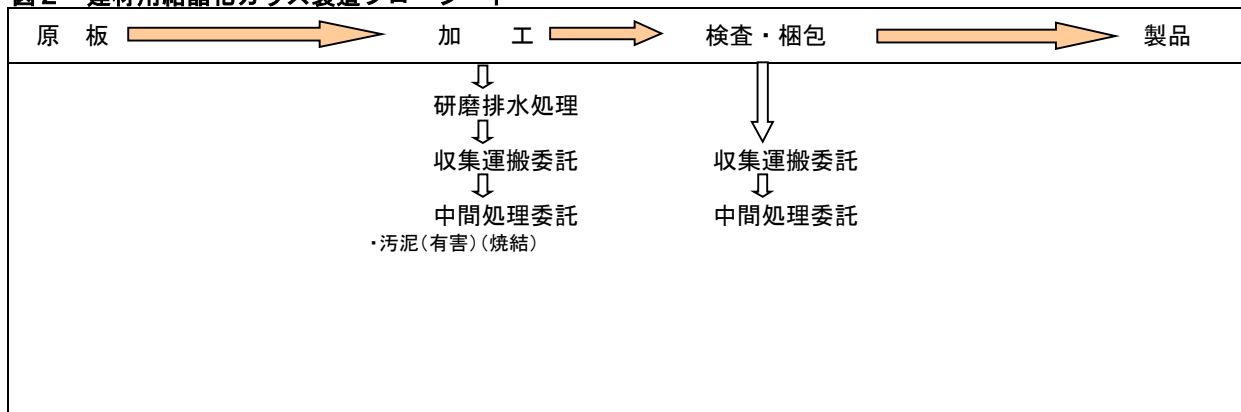
図2 建材用結晶化ガラス製造フローシート
