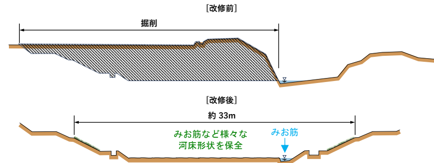
真野川横断面 (2)家田橋上流(河口から約2.7km)
