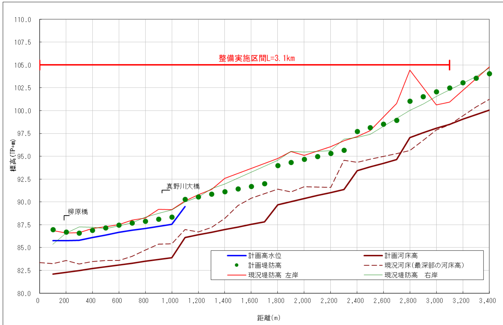
図 真野川縦断面
