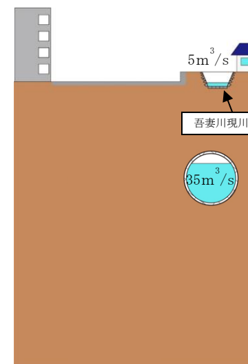
吾妻川横断面図 滋賀県庁前(河口から約 0.8km)
