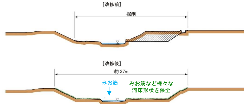
真野川横断面 (1)真野川大橋下流(河口から約0.7km)
