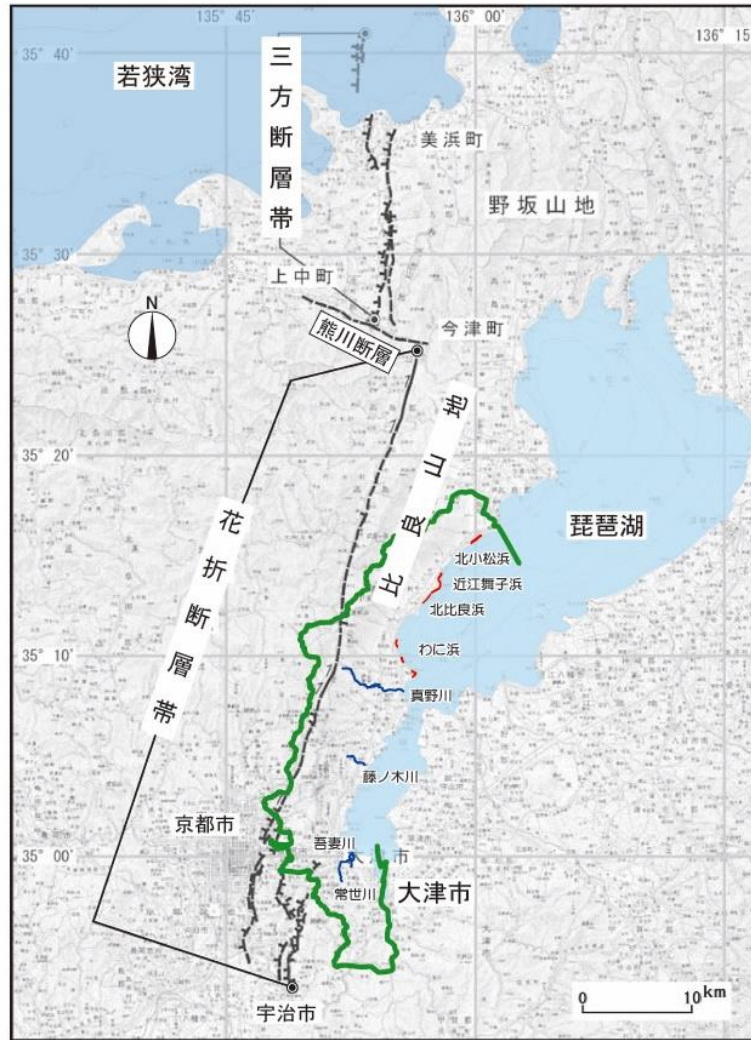
図 花折断層帯位置図
