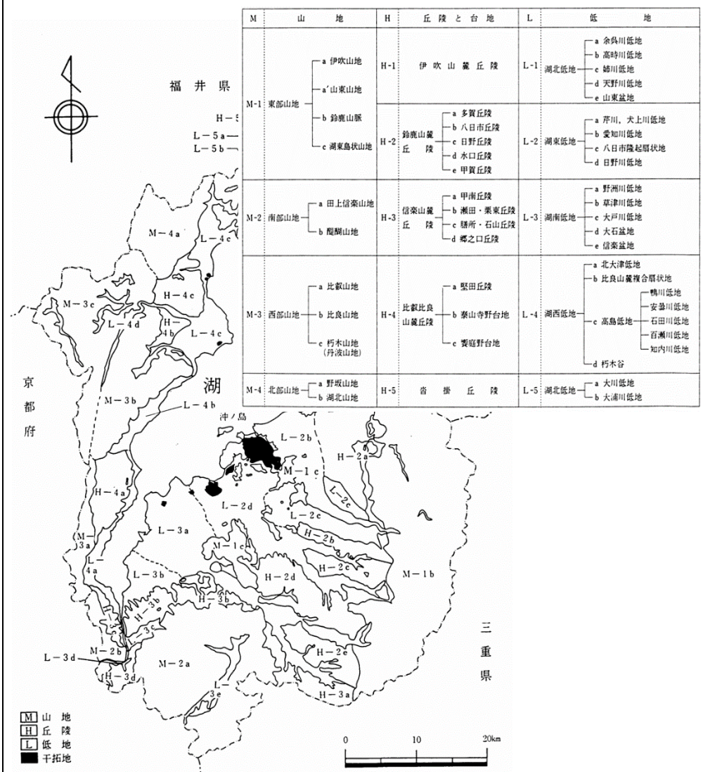
図 滋賀県地形区分図
