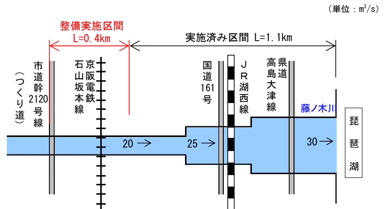
藤ノ木川 計画流量配分図
