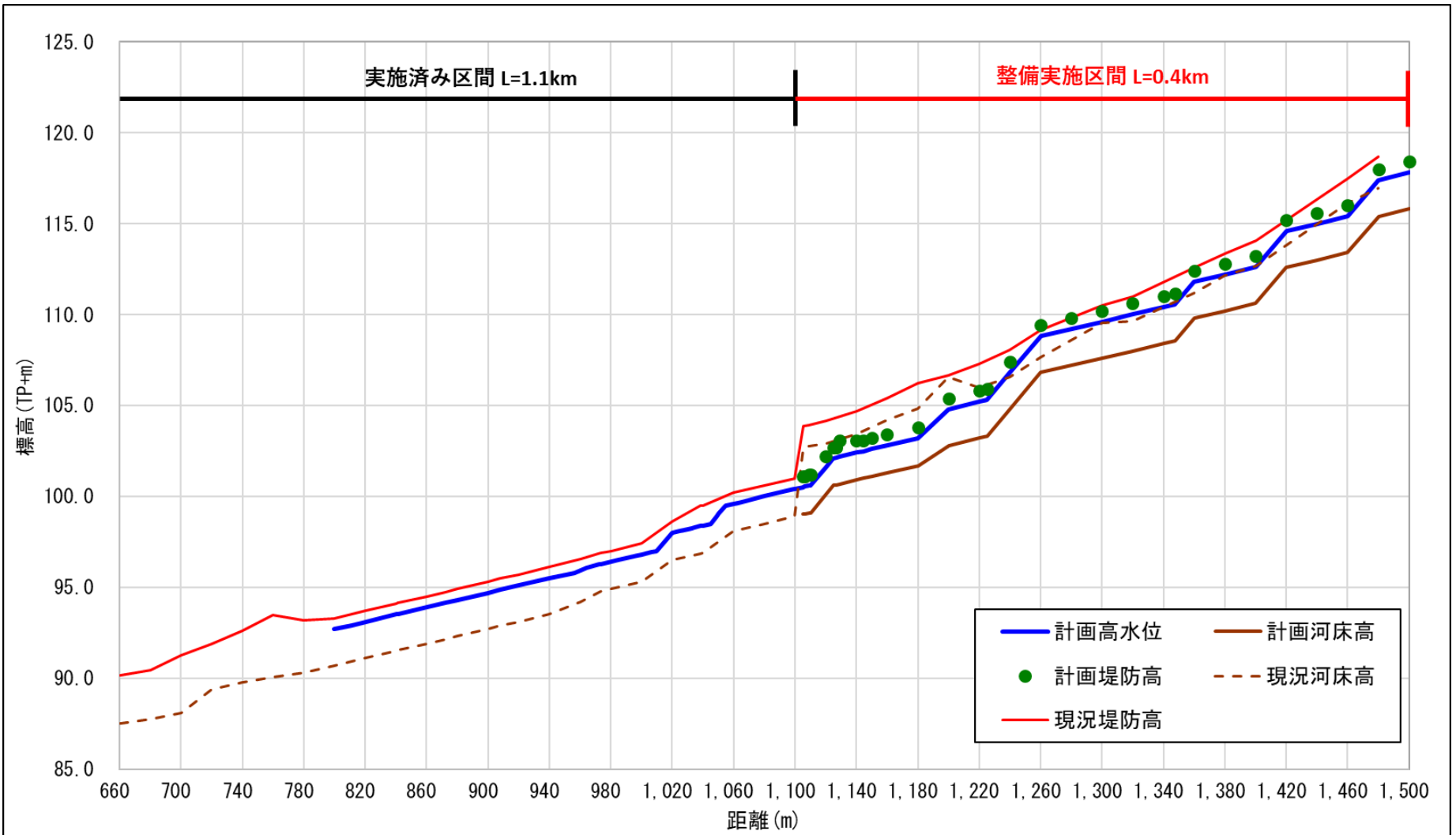
図 藤ノ木川縦断面
