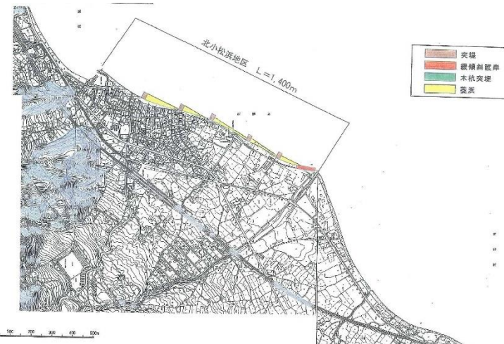
図 北小松浜地区計画平面図
