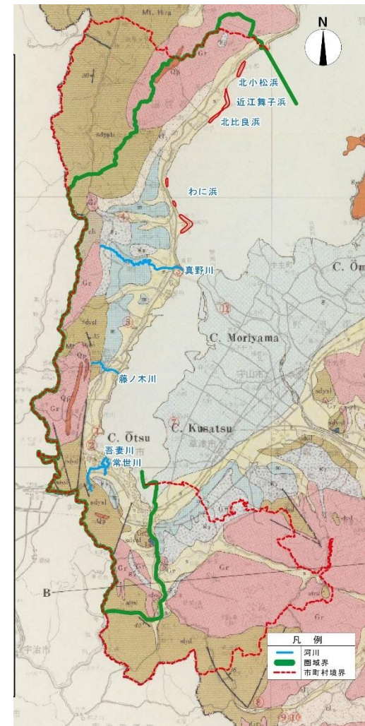
図 志賀・大津圏域地質図
