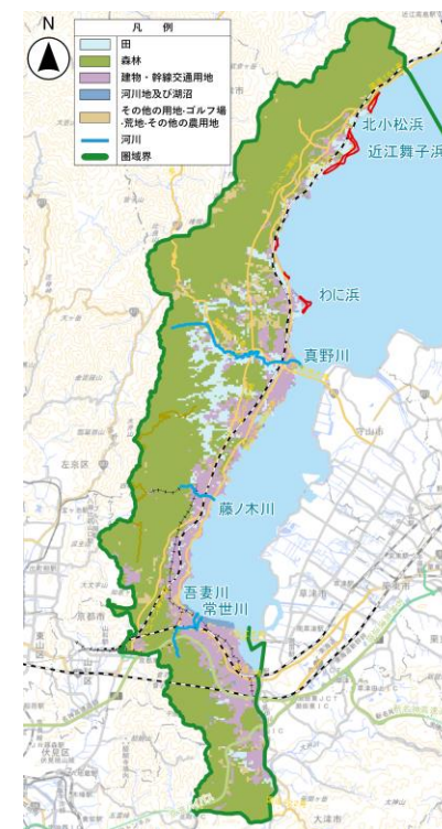
図 志賀・大津圏域土地利用図(R3)
