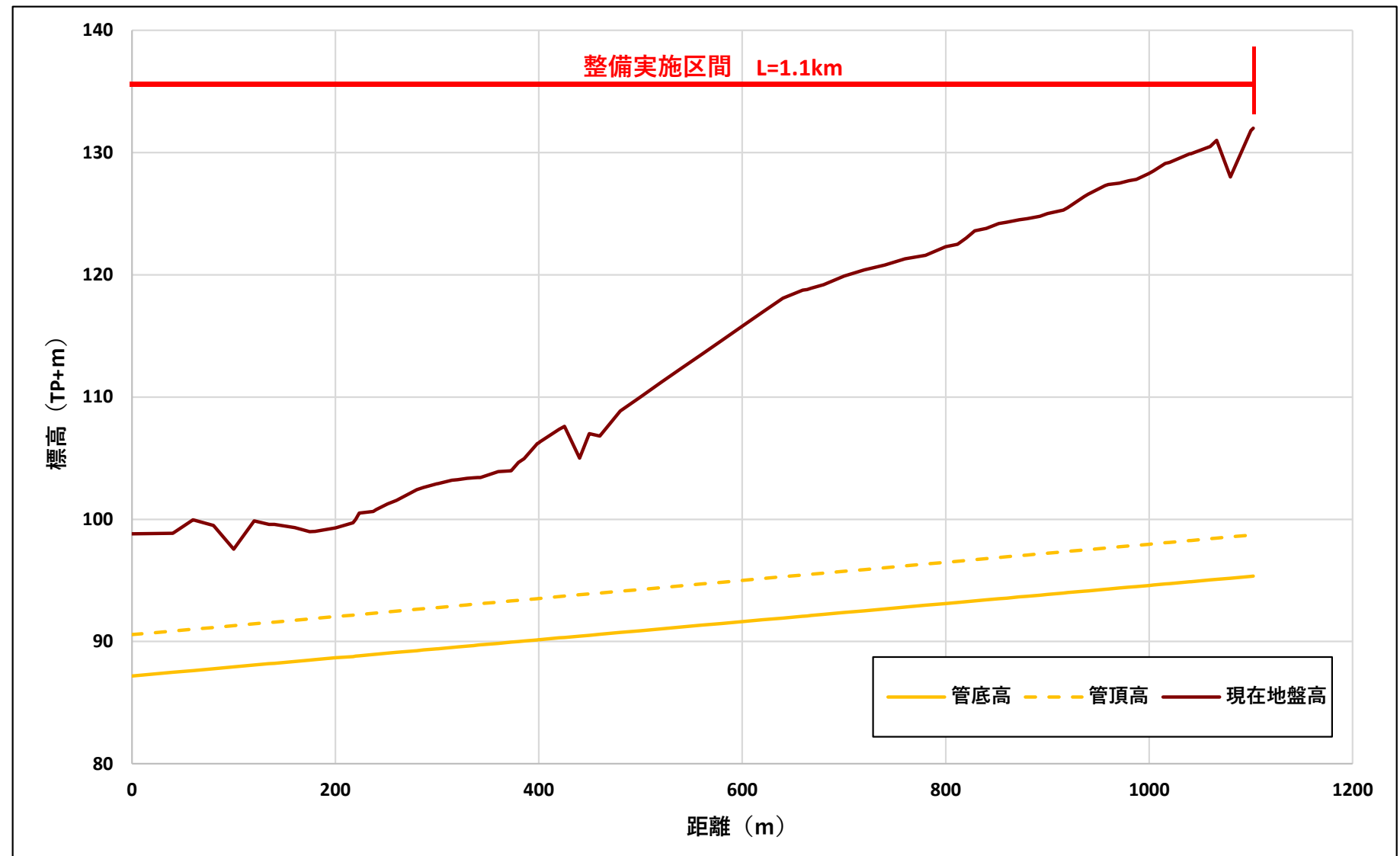
図 吾妻川縦断面
