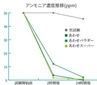
図 2 アンモニア濃度推移
