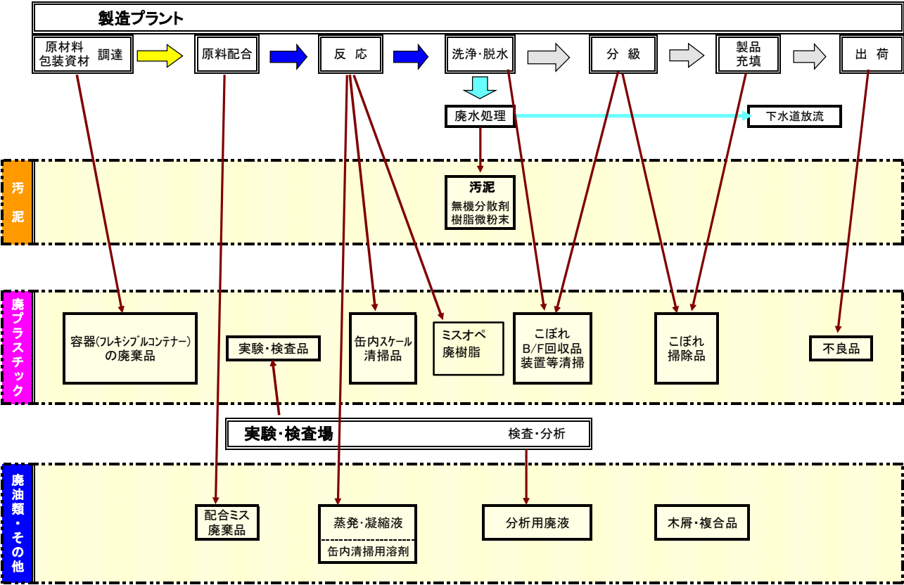
産業廃棄物の発生フロー
