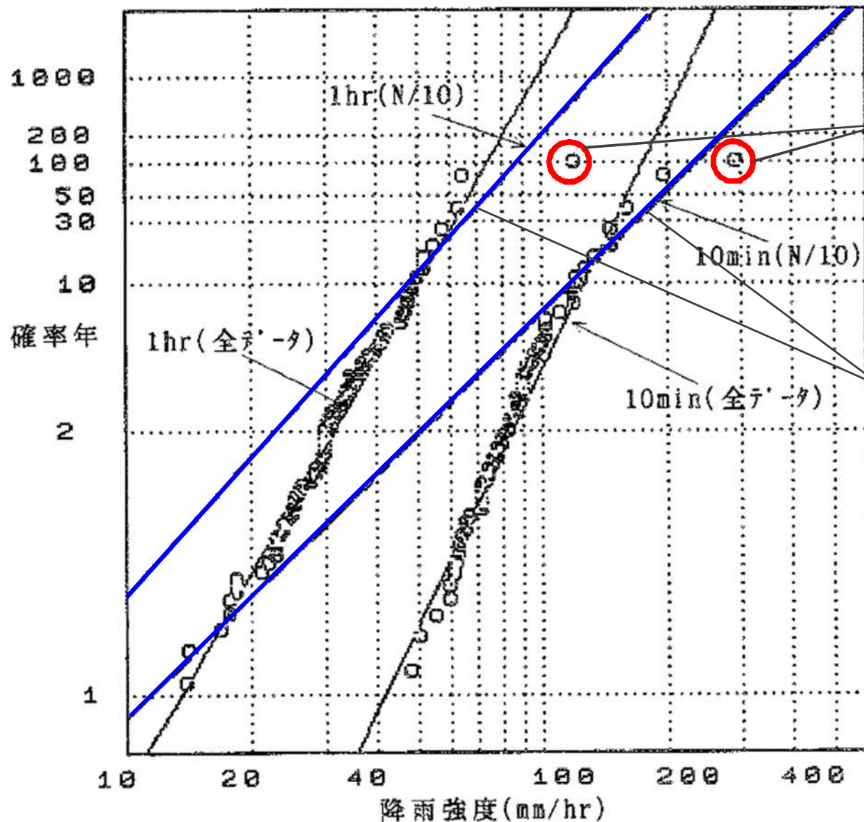
図-3 確率降雨強度(1hr,10min)
