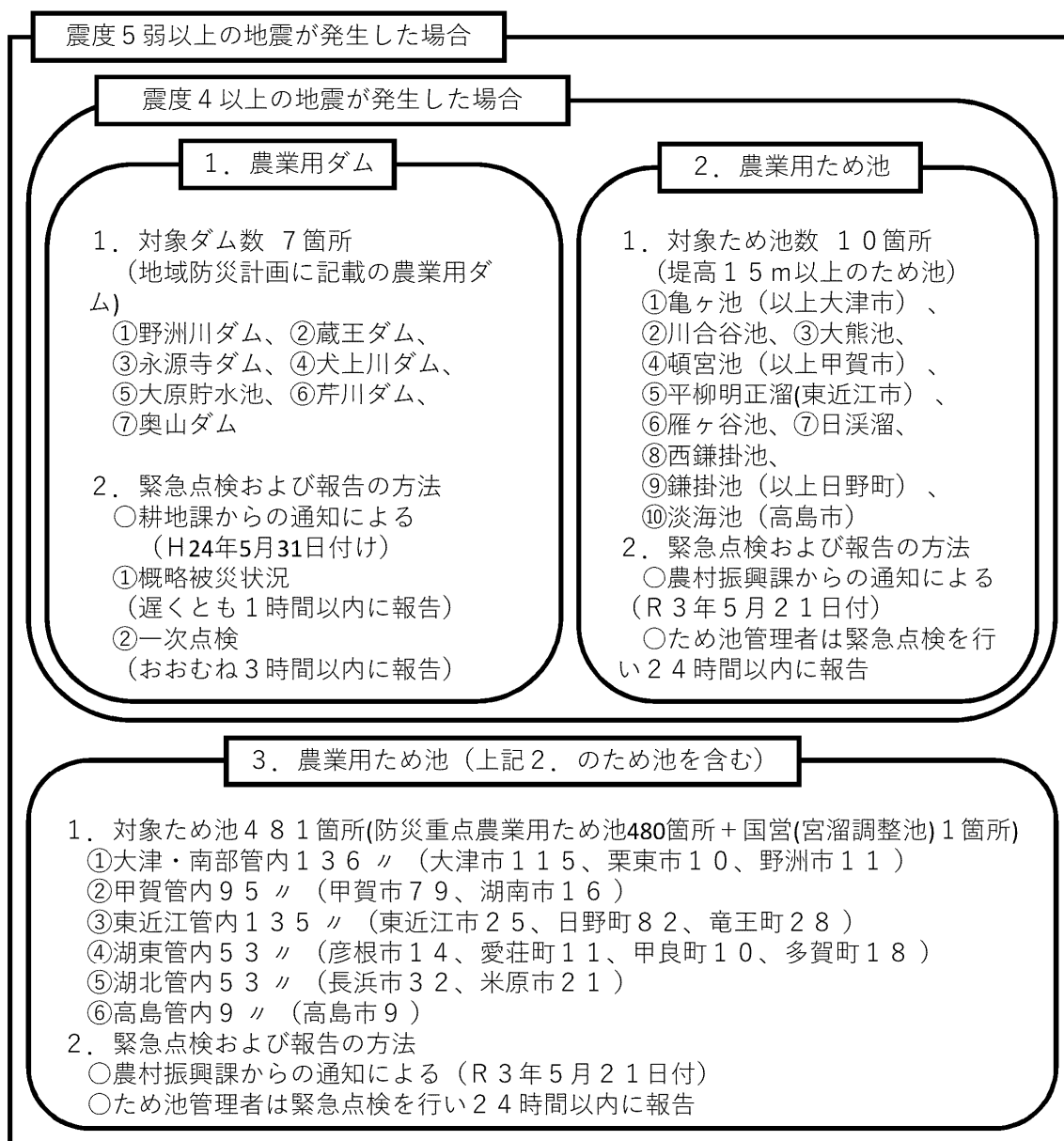
図VI-6 地震発生時における農業用ダム・ため池の点検および報告の区分 (R4.4)
