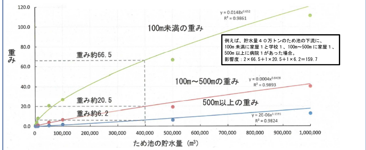
図V-3 ため池の貯水量と浸水想定区域の家屋や公共施設等との距離に応じた影響の数値化 （防災重点ため池における対策の進め方(国通知 H31.3)）
