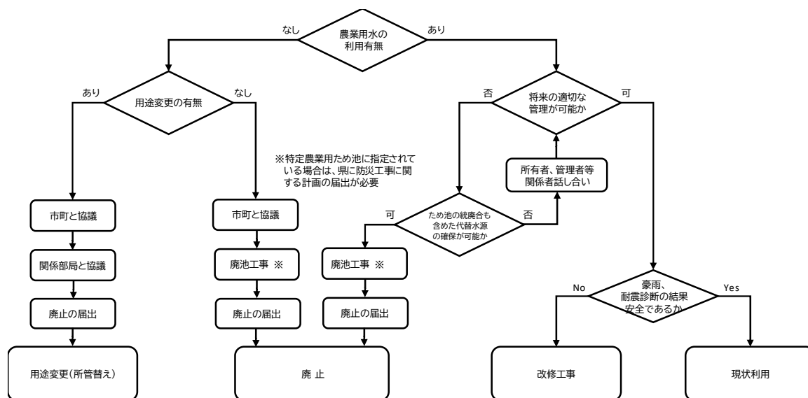
図V-5 ため池の廃池に至るプロセス（ため池管理者等が明らかな場合を想定した例）
