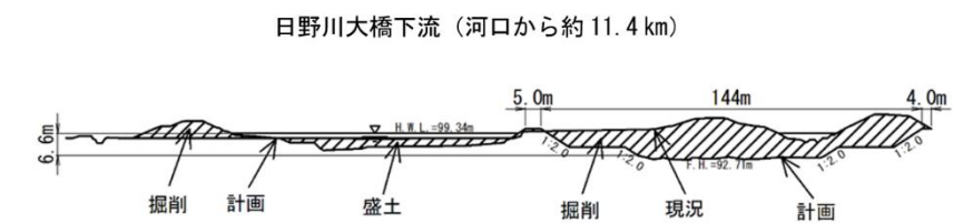
横断図
