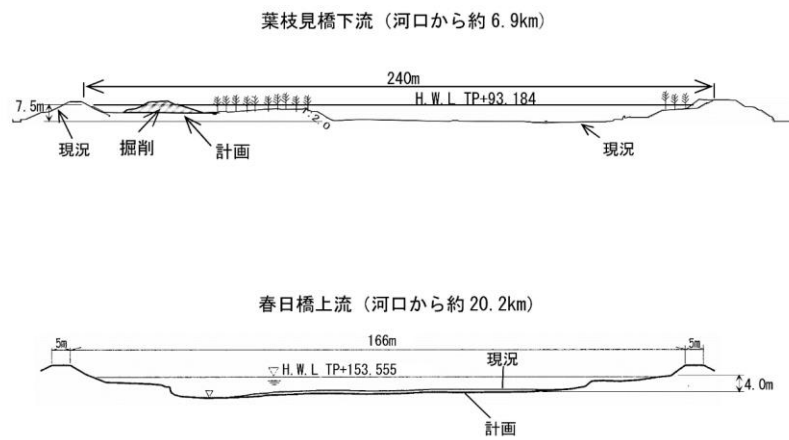
横断面図
