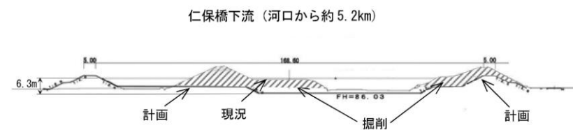
横断図
