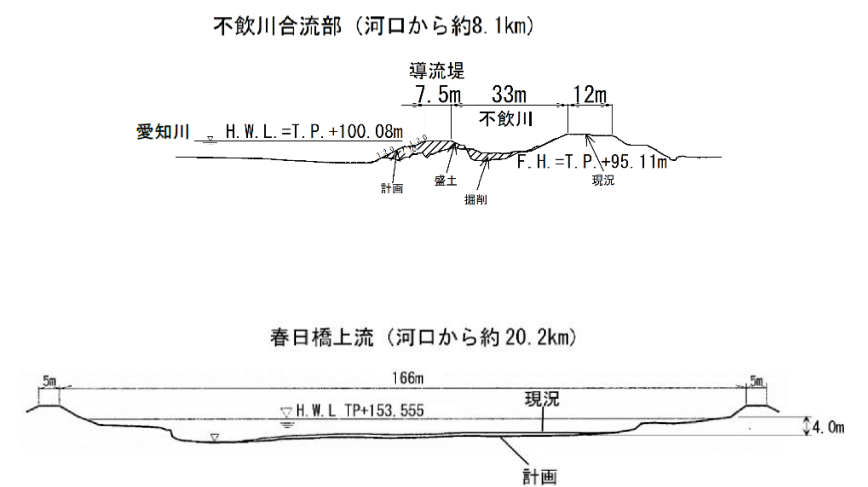
横断面図
