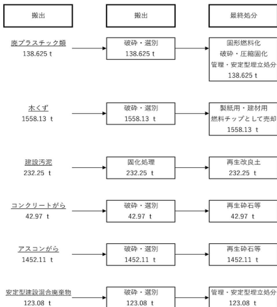
産業廃棄物処理工程表
