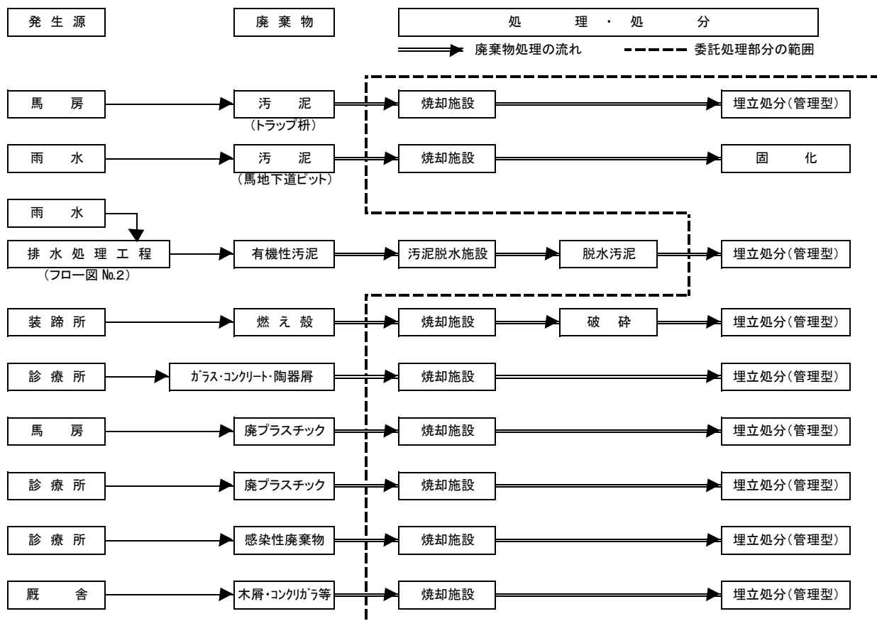
廃棄物処理フロー図(現状) No.1
