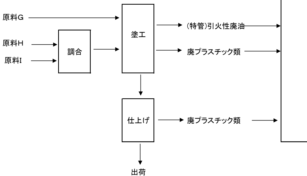
フィルム製造フロー図
