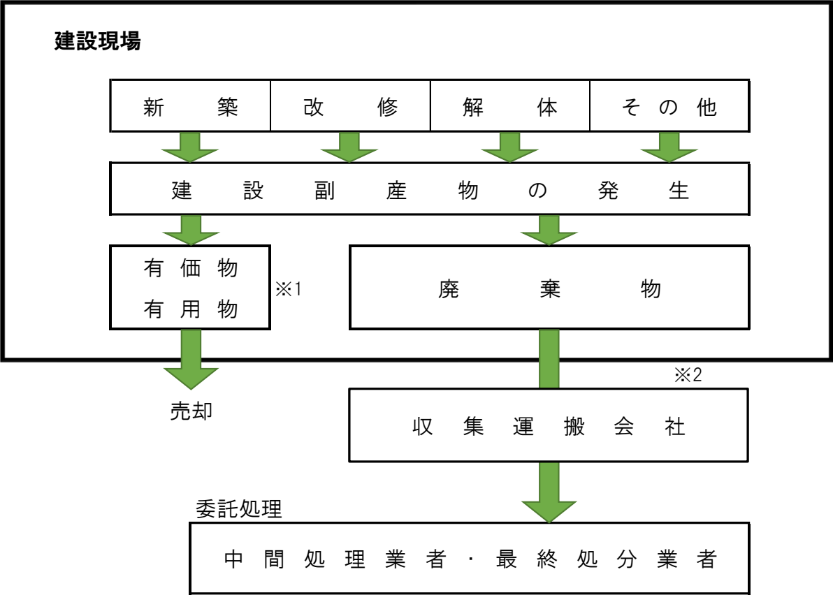
別紙1 産業廃棄物の一連の処理工程図
