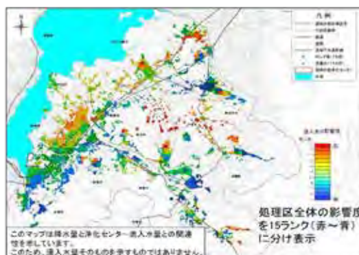
図2 取組対策例：不明水影響度マップ
