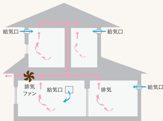
24時間換気システムの一例
