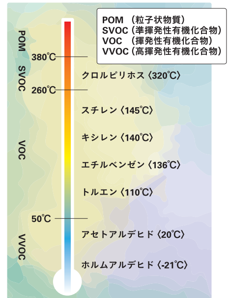
図1 揮発性の有機化合物の沸点と分類
