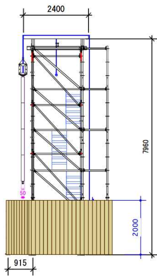
【側面図】
