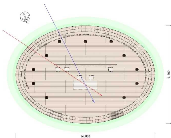
【平面図】
