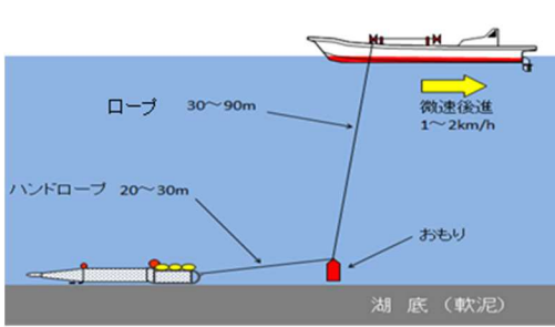
図3 そりネット曳網方法
