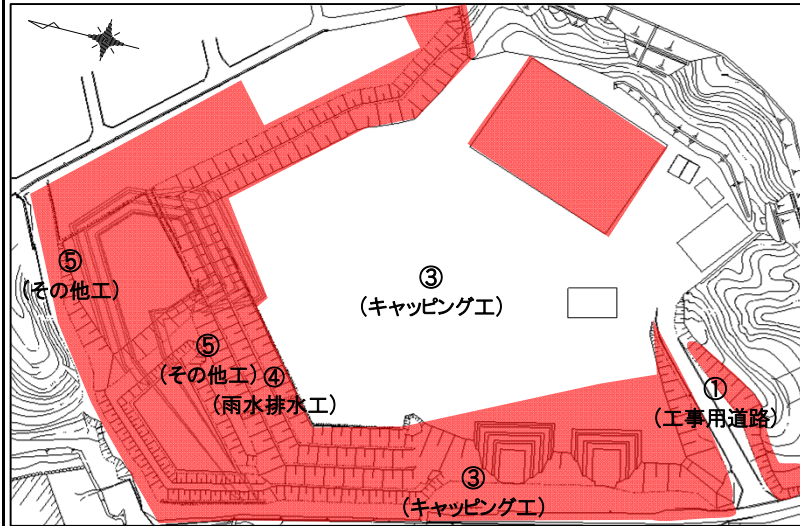
① 工事用進入路 法面部モルタル吹付を行っています。
