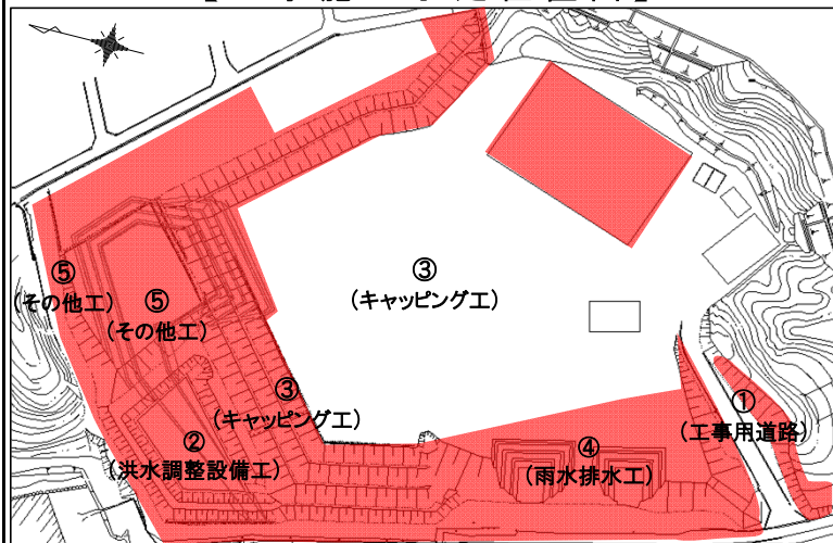
【工事施工予定位置図】
