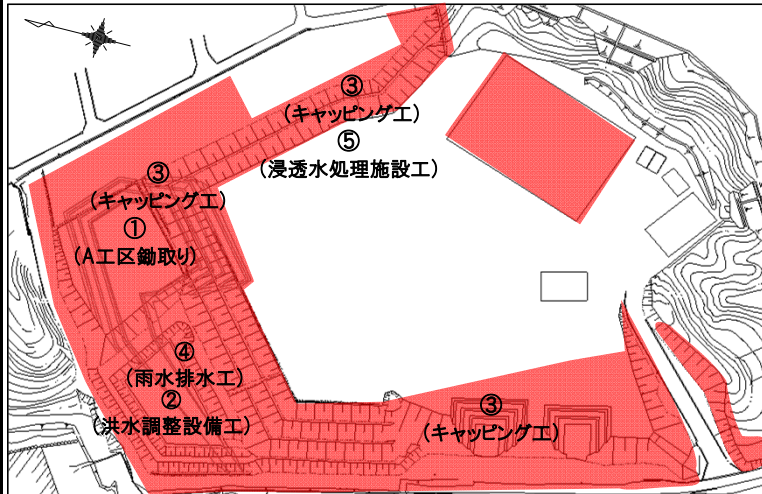
③ キャッピング工 北尾団地側法面モルタル吹付を行っています。
