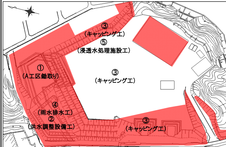
③ キャッピング工 北尾団地側法面ラス網のアンカーピン打設を行っています。
