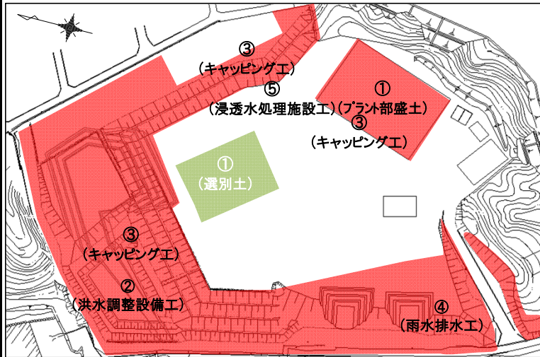
③ キャッピング工 B工区法面覆土整形を行っています。
