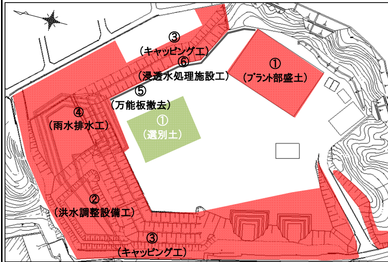
② 洪水調整設備工 セメント改良土工を行っています。
