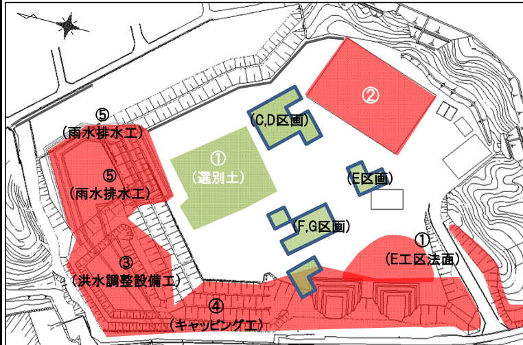
① 選別土仮置・盛土工
