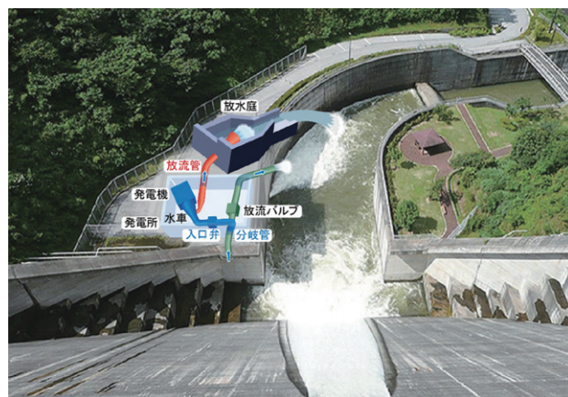
県営姉川ダムにおける水力発電の仕組み
