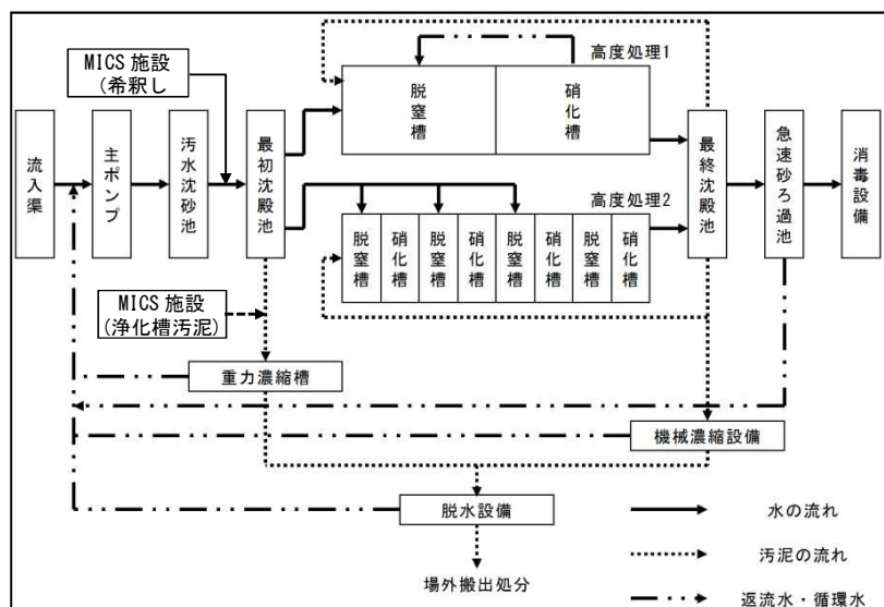
図3 高島浄化センター処理フロー（事業計画（平成30年度））
